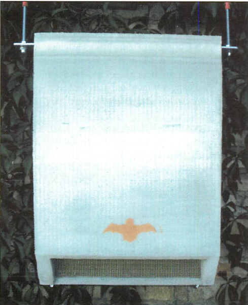
Abb. 3. Starkfrosthabitat mit integrierter Tragschiene für die Deckenmontage.
