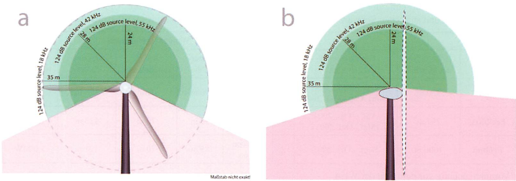
Abb. 1. Erfassungsbereich der Batcorder auf den WEA und Auswirkung des Schallschattens der Gondel auf den akustisch überwachten Bereich von frontal (a) und lateral (b). In den Abbildungen sind außerdem die Detektionsreichweiten für verschiedene Fledermausarten eingetragen (70 % Luftfeuchte, 10° C, Erfassungsschwelle 5 % der Maximalamplitude). Die angenommene Rufflautstärke von 124 dB SPL in 10 cm Abstand liegt etwas unter dem bekannten Maximum für die einzelnen Arten (HOLDERIED & VON HELVERSEN 2003).
