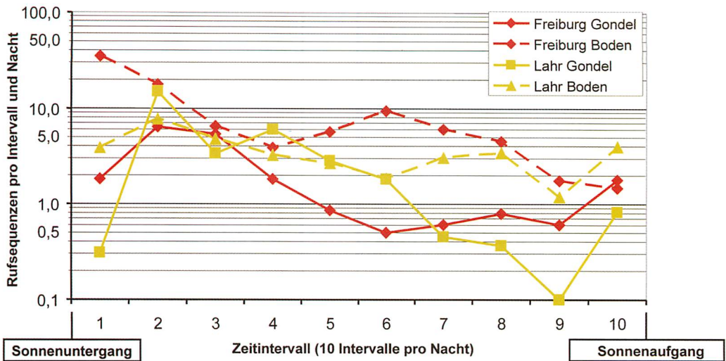
Abb. 3. Anzahl aller an der WEA-Gondel und am Boden registrierter Ortungsrufsequenzen je Nachtintervall und Nacht (Standort Freiburg 2004 und Lahr 2005 – Ordinate logarithmuskaliert). Ein Zeitintervall entspricht jeweils einem Zehntel der Untersuchungsnacht. Intervalllänge zwischen 50 und 84 min. Daten gemittelt pro Intervall für Freiburg Gondel und Boden: 10 bis 12 Nächte, Lahr Gondel: 10 bis 11 Nächte, Lahr Boden: 22 bis 29 Nächte.
