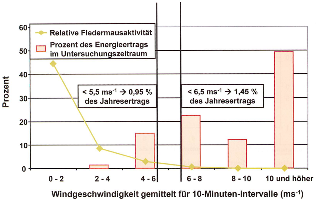
Abb. 4. Fledermausaktivität an der WEA-Gondel und Ertrag in Abhängigkeit von der Windgeschwindigkeit. Gezeigt ist der Energieertrag und die Fledermausaktivität während der Untersuchungszeiten in Abhängigkeit von der Windgeschwindigkeit (gemittelt für 10-min-Intervalle). Die relative Aktivität ist angegeben als prozentualer Anteil von 10-min-Intervallen mit Fledermausaktivität von insgesamt untersuchten 10-min-Intervallen pro Windgeschwindigkeitsklasse ( n = 770 insgesamt mit Batcordern untersuchte 10-min-Intervalle, davon 46 Intervalle mit Fledermausregistrierung). Senkrechte Striche markieren mögliche „fledermausverträgliche“ Anlaufgeschwindigkeiten der WEA von 5,5 oder 6,5 \text{ ms}^{-1} . Die Boxen geben jeweils die auf den Gesamt-Jahresertrag bezogenen Einbußen für die vorgeschlagenen Anlaufgeschwindigkeiten (höhere Anlaufgeschwindigkeiten von Anfang Juli bis Ende September, nur nachts - Standort Freiburg im Jahr 2004) an.
