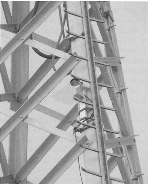
Abb. 2. Anbringen des Mikrofons und des Spiegels sowie des Detektors und der Stromversorgung in einem PU-Rohr am Mast. Microphone with mirror as well as detector and power supply in a tube fixed to the mast.
