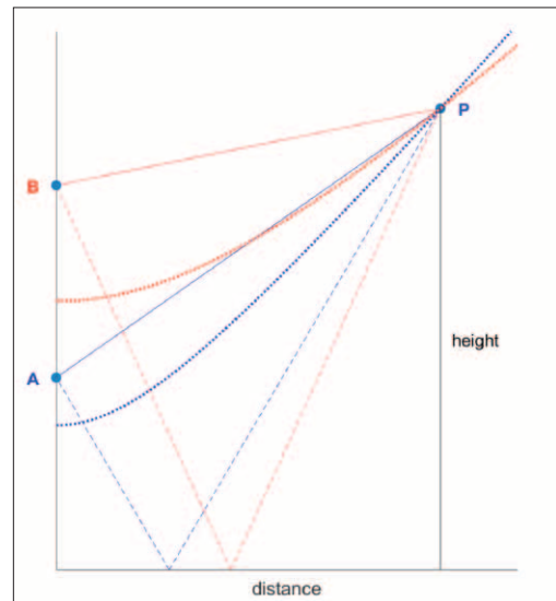
Abb. 1: Zwei Ultraschallmikrofone A und B, die senkrecht übereinander über der Wasseroberfläche angebracht sind, nehmen die Rufe der Fledermaus P über den direkten Weg (durchgezogene Linien) und als Reflexion (gestrichelte Linien) auf. Gepunktet sind die Linien konstanter Zeitdifferenz.
