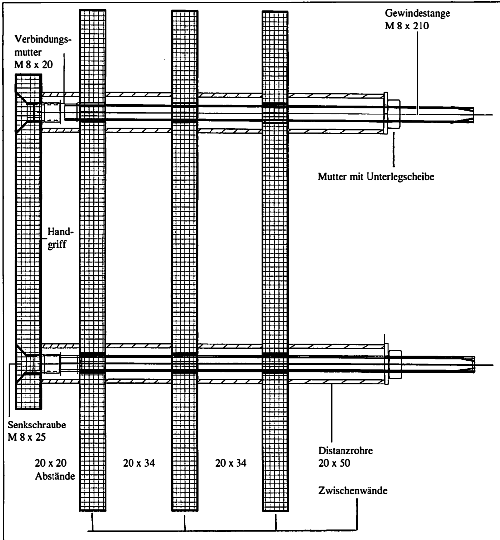
Abb. 1. Skizze für den umgebauten und herausnehmbaren Einsatz in die Fledermaus-Großraumhöhle 1FW der Fa. Schwegler. Zeichnung: CHR. KUTHE
