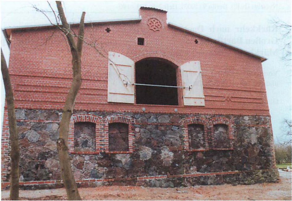
Abb. 1. Westgiebel des ehemaligen Stallgebäudes in Julianenhof mit einer ehemals zur Beschickung des Bodens dienenden Öffnung. Der gesamte Giebel oberhalb des Feldsteinsockels wurde erneuert, die große Öffnung mit neuen Flügeltüren versehen. Aufn.: M. Kretschmer
