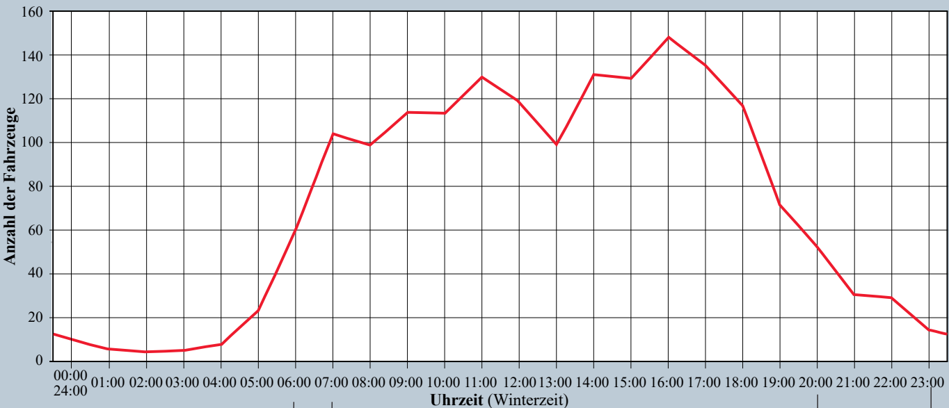
Absenkbetrieb in den Dunkelstunden abhängig vom Verkehrsaufkommen
