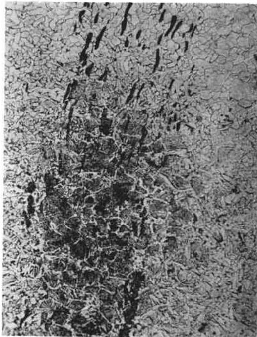
10 Mikrogefüge, 65:1
