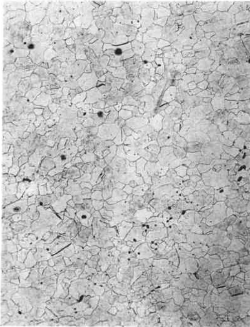
9 Mikrogefüge, 65:1
