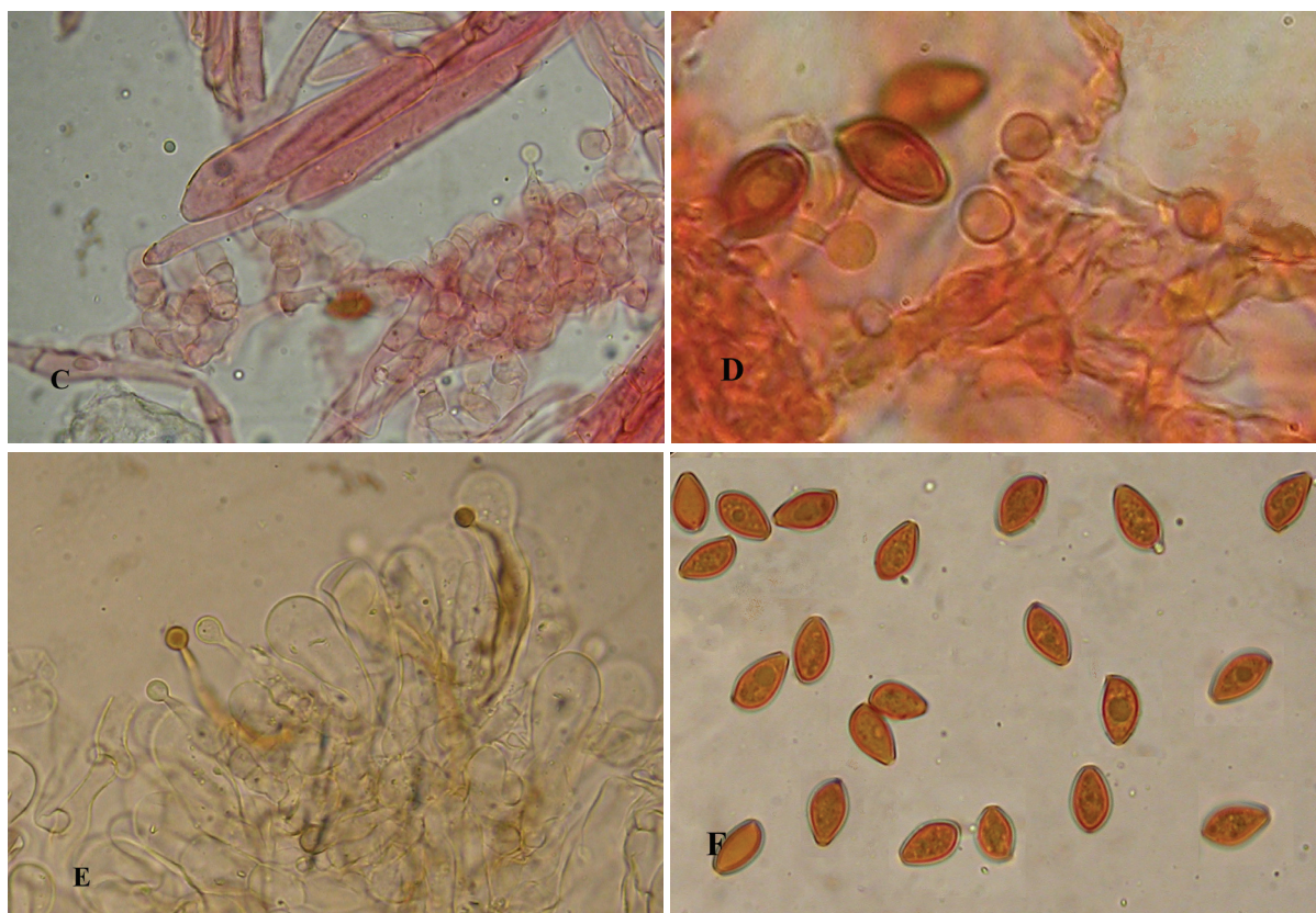
Fig. 2. Conocybe volvicystidiata , holotype, caracteres microscopiques, C caulocystides dans le haut du stipe (poils et une seule caulocystide lecytiforme), D pileipellis avec nombreuses pileocystides lecytiformes, E strate extérieure de la volve avec plusieurs cystides lecytiformes, F spores. – Phot. M. BROUSSAL
