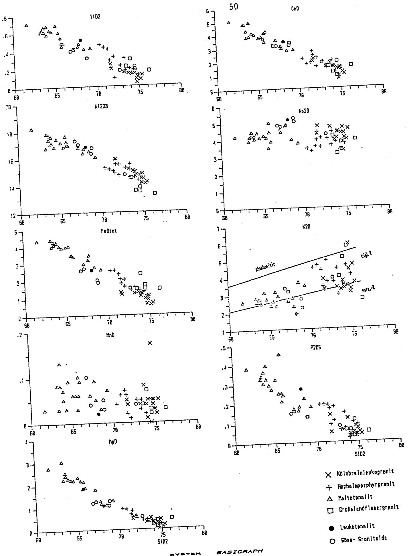
Abb. 26: Hauptelementvariation der Zentralgneise (Harker-Diagramme) aus: MARSCHALLINGER & HOLUB 1989
