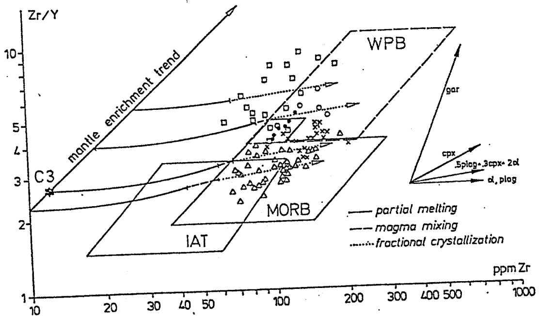
Abb. 5: Zr/Y vs. Zr- Diagramm. Die ophiolitischen Basalte fallen ins MORB-Feld, einige Eklogite, die Fuscher Metabasite und die Amphibolite aus den westlichen Hohen Tauern plotten im WPB (within-plate-basalt)-Feld, Zug III- Magmen in den Grenzbereich. Die meisten Eklogite zeigen typische WPB- Zr/Y- Verhältnisse, jedoch niedrigere Zr- Gehalte. C3: C3-Chondrit nach PEARCE&NORRY (1979).
