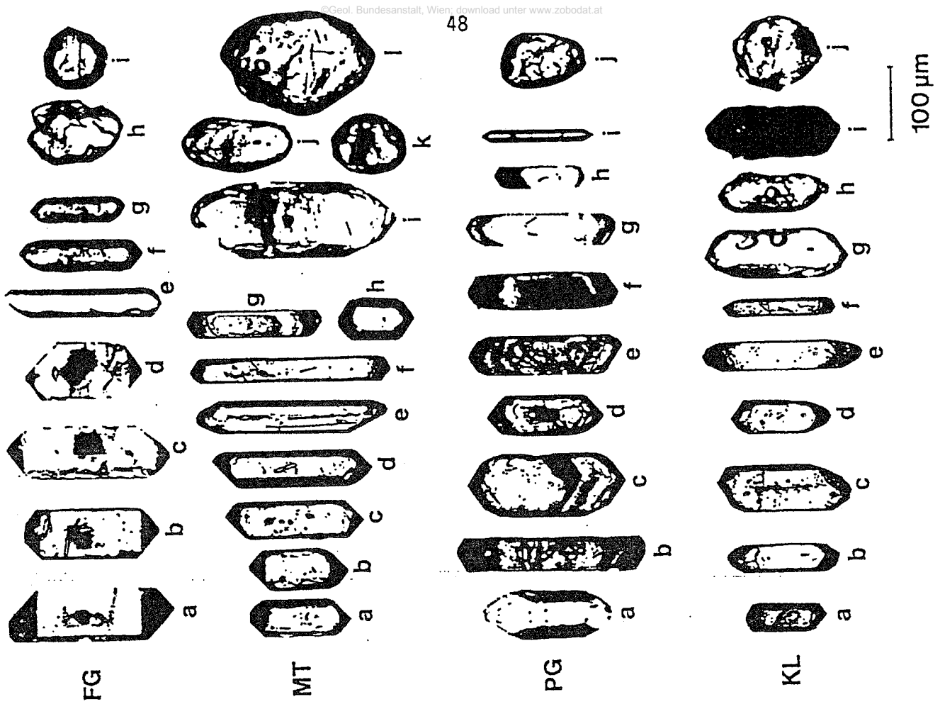
Abb. 24: Charakteristische Zirkontypen aus alkristallinen Mikrofiltration und Zentralgneisen des oberen Malaitales
