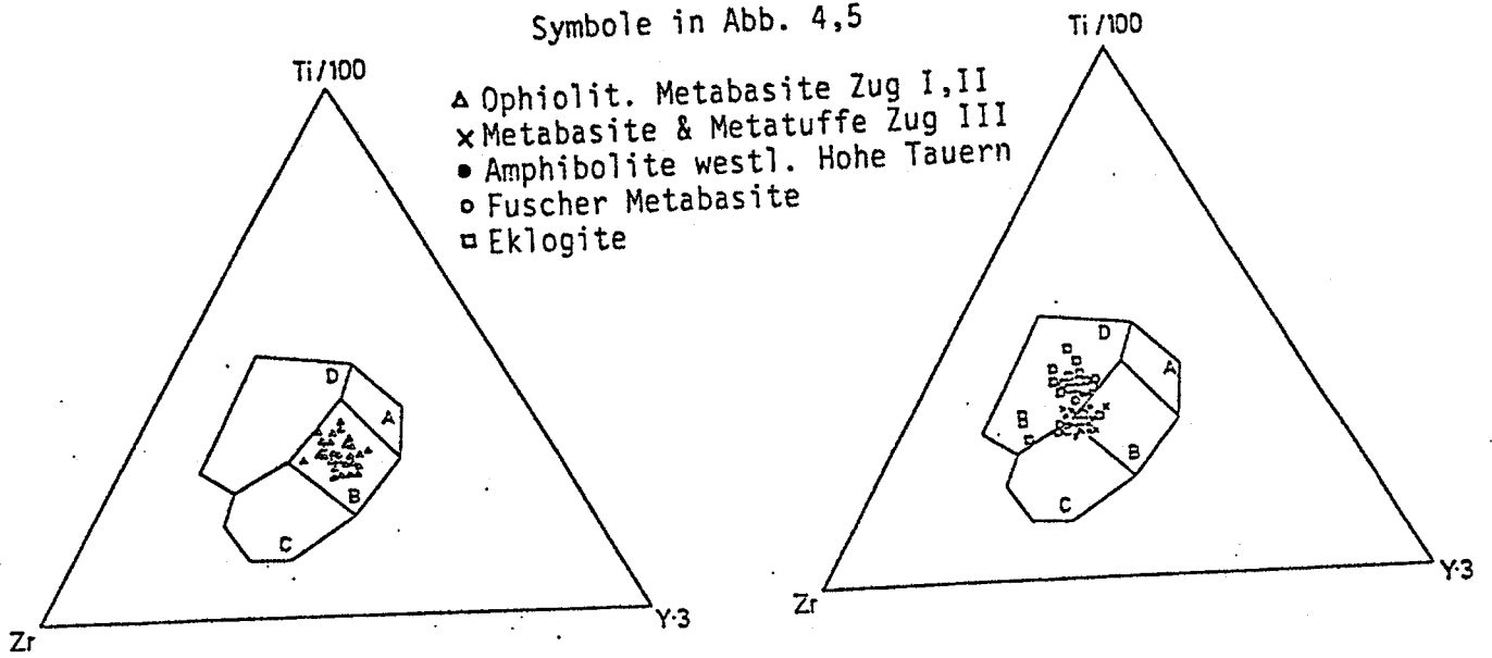
Abb. 4: Ti/100-Zr-Y*3 Dreiecke nach PEARCE & CANN (1973). Ozeanbodenbasalte plotten in Feld B, Within-plate-Basalte in Feld D, low-K-Tholeiite in Feld A&B, Kalkalkalibasalte in Felder B&C. Die ophiolitischen Metabasite fallen eindeutig ins MORB-Feld B. Die meisten Eklogite plotten im Feld D - wie die Fuscher Metabasite - beide Gruppen überlappen etwas die Felder B&C. Die Amphibolite aus den westlichen Hohen Tauern und die Magmen von Zug III fallen auf den Grenzbereich zwischen Feld B&D.
