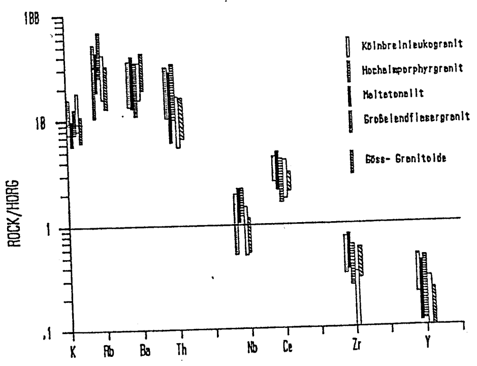
Abb. 29: Variation der Spurenelementgehalte der Zentralnase im HORG- normierten geochemischen Pattern
