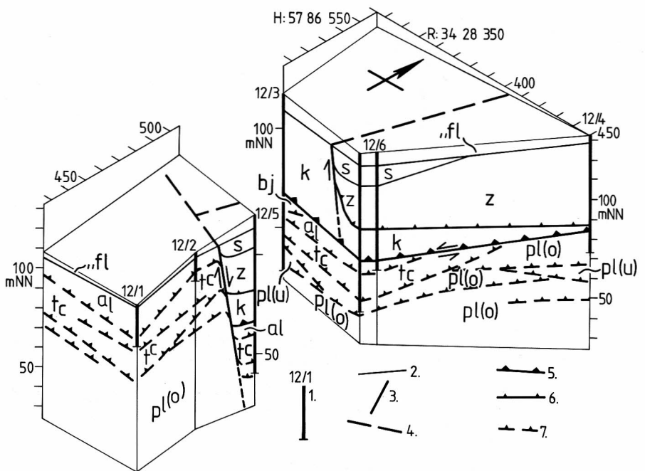
Abb. 2 Blockbild (isometrische Projektion) vom N-Hang des Silberberges mit den Bohrungen 12/1 bis 12/6, z. T. hypothetisch (grau: Silberberg-Großheide-Scholle).
