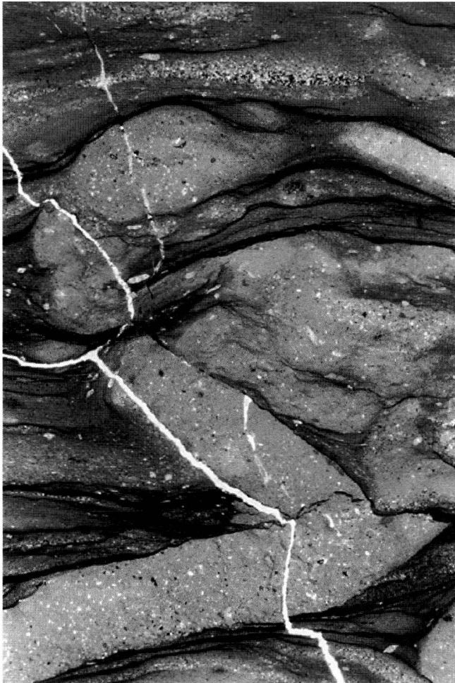
Abb. 5 Mikrofaziestyp C; Mauerstein K12. Dünnschliff-Foto, Vergrößerung 6 ×.
