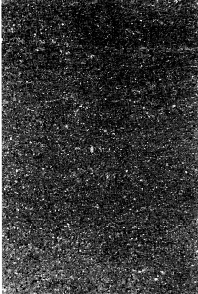
Abb. 4 Mikrofaziestyp B; Mauerstein K8. Dünnschliff-Foto, Vergrößerung 12 x.
