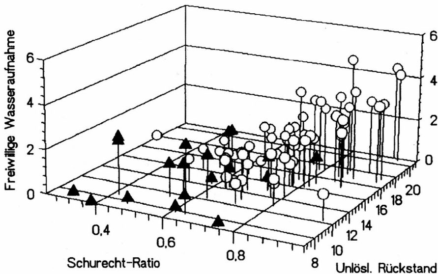
Abb. 10 Diagramm der Korrelation zwischen der Schurecht-Ratio, der freiwilligen Wasseraufnahme (in Vol.-%) und dem Gehalt an salzsäureunlöslichem Rückstand (in Gew.-%) in den Mauersteinen des Schwesternhauses. Zeichenerklärung: ▲ = Mikrofaziestypen A + B; ○ = Mikrofaziestypen C-E.
