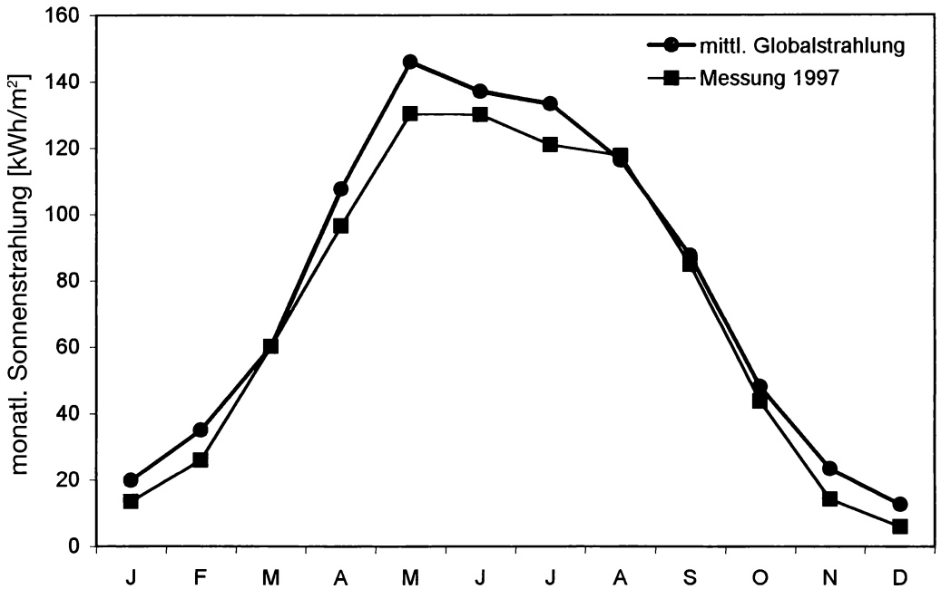
Abb. 3: Monatliche Sonnenstrahlung 1997 ( \text{kWh/m}^2 ) verglichen mit der 1979–1982 gemessenen Globalstrahlung.
