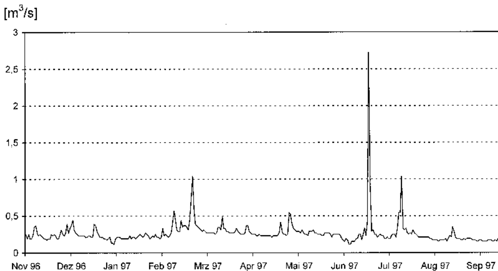
Abb. 2: Abfluß des Belmer Bachs am Pegel Gretesch (M3, 800 m vor Mündung). Datenquelle: StAWA Cloppenburg.
