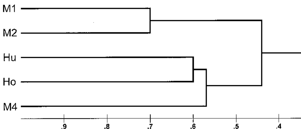
Abb. 10: Dendrogramm der UPGMA-Linkage der Sørensen-Indizes (aus Rohdaten, Cophenetic Coefficient = 0,9535). Berechnet aus den Probenahmen 1997.
