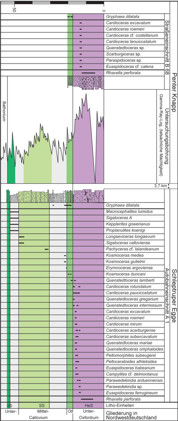
Abb. 7: Korrelation der Aufschlüsse Schleptruper Egge und Penter Knapp sowie dem Gamma-Ray-Log der UB Penter Knapp unter Berücksichtigung der Ammoniten
