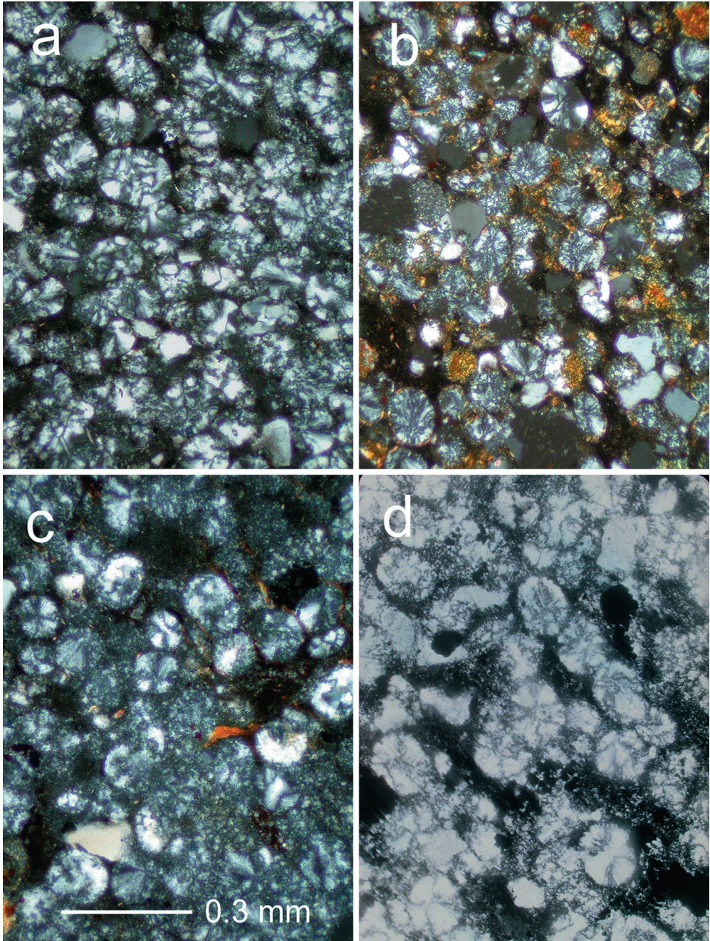
Abb. 3: Dünnschliffe von Spiculiten mit Rhaxella perforata Hinde
