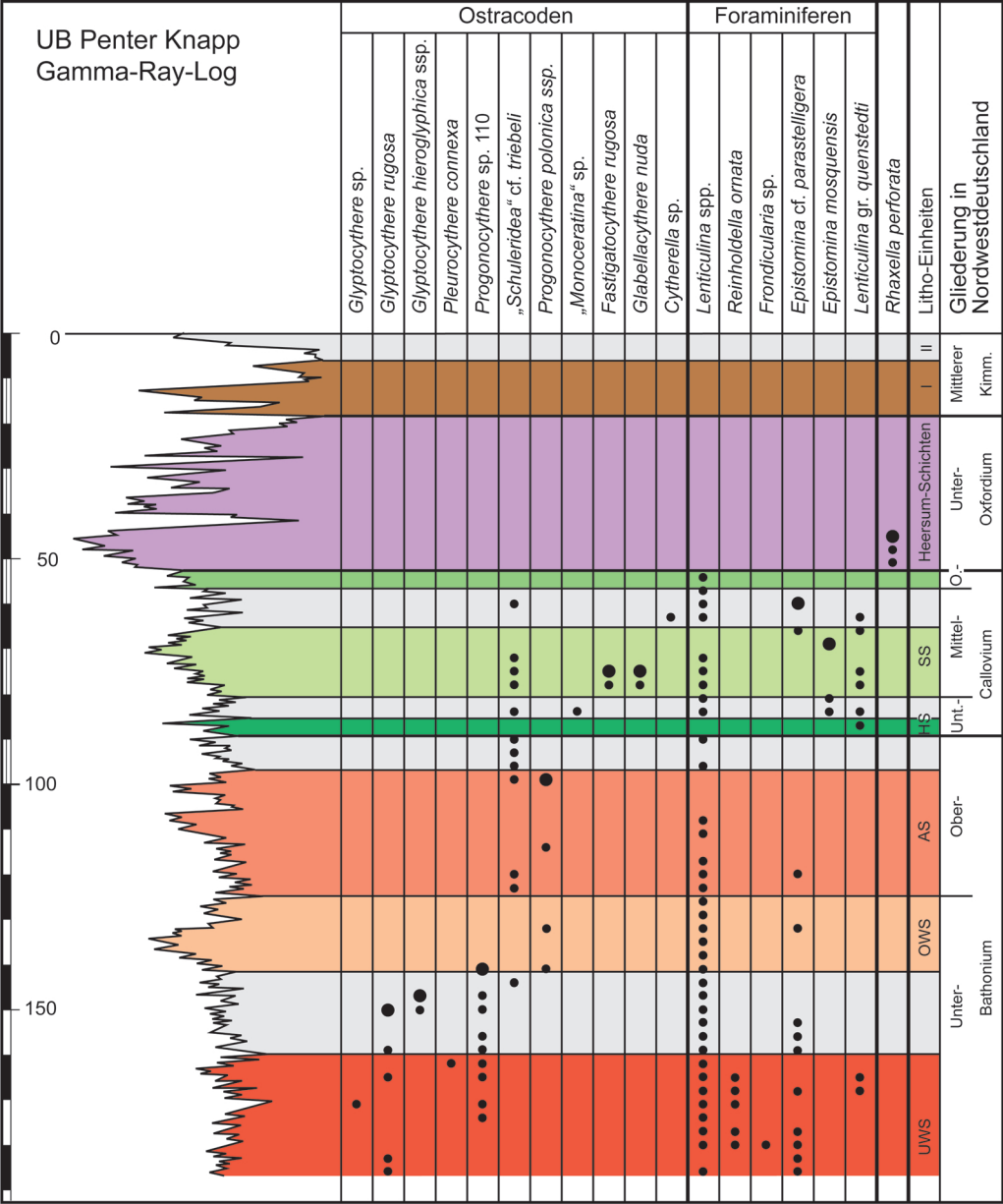
Abb. 8: Gamma-Ray-Log und Fauna der UB Penter Knapp
