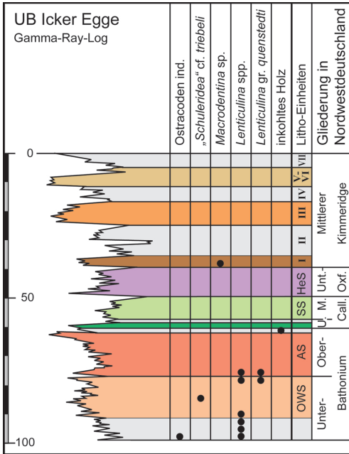
Abb. 5: Gamma-Ray-Log und Mikrofauna der UB Icker Egge
