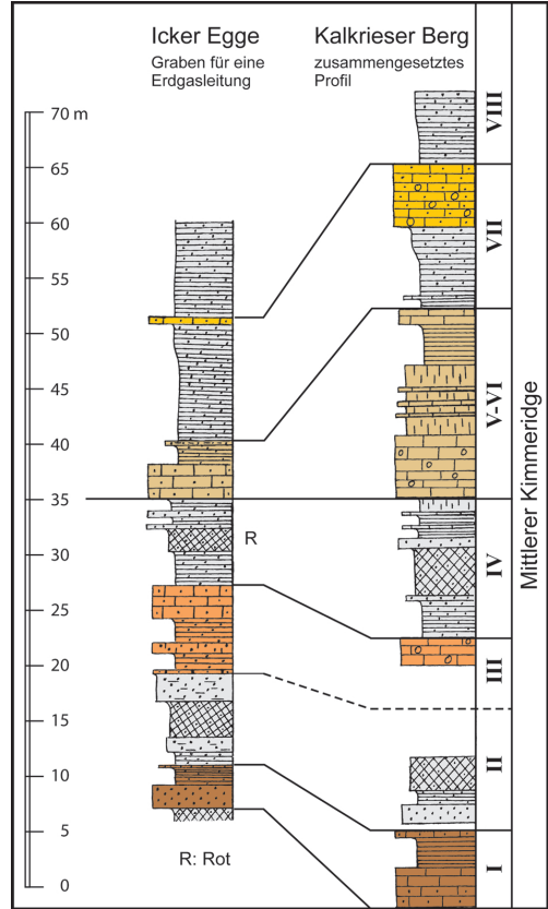
Abb. 4: Schichtenfolge des tiefen Mittel-Kimmeridge (MK I–VII) im Graben für eine Erdgasleitung an der Icker Egge und im Nordteil des Kalkrieser Berges
