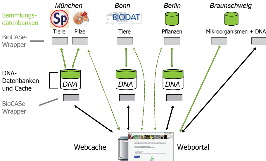
Abb. 1: Datenfluss im DNA-Bank-Netzwerk. Die Datenarchitektur basiert auf der Infrastruktur von GBIF. Beleginformationen (grüne Linien) werden über BioCASe-Wrappers (graue Boxen) an die DNA-Module und das Webportal übertragen. Die Wrapper für die Belegdaten sind dieselben, die auch GBIF benutzt. Über eine zusätzliche BioCASe-Wrappers-Installation auf den DNA-Modulen und der Datenbank in Braunschweig werden die DNA-Daten (schwarze Linien) an den Webcache und das Webportal übertragen. Das Webportal ist dadurch in der Lage, sowohl die Beleg- als auch die DNA-Daten „live“ (Original-Daten aus den jeweiligen Datenbanken) anzuzeigen.
