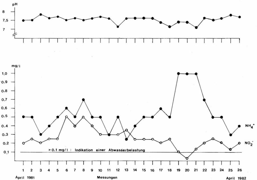
Abb. 3: Jahresgang des pH-Wertes, des Nitrits (NO 2 - ) und des Ammoniums (NH 4 + ) an Probestelle P 7. Indikationswert der Abwasserbelastung nach SCHWOERBEL 1980a.
