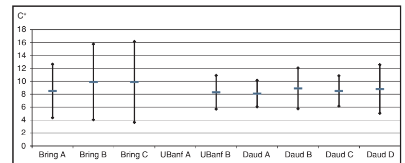
Abb. 11: Jahresmittel und Spanne \Delta t^{\circ}\text{C} des mittleren Temperaturmaximums und -minimums.
