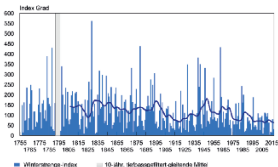
Abb. 5: Winterkältesummen in Mannheim der Winter 1755/56 bis 2017/18.
