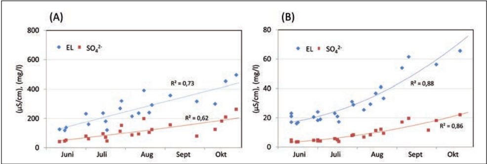
Abb. 5: Elektrische Leitfähigkeit (EL, \mu\text{S}/\text{cm} ) und Sulfatkonzentration [\text{SO}_4]^{2-} ( \text{mg}/\text{l} ) im Abfluss an den Stellen HK-P (A) und HK-Z (B). Einzelproben Juni–Oktober, 2007–2012, wurden zu einer Serie zusammengefügt.
