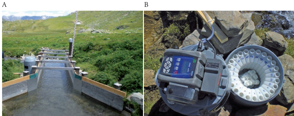
Abb. 2: Pegel des Hydrographischen Dienstes (Land Tirol) am Hohebenkarbach auf 2.220 m Höhe (A), Automatischer Probesammler (B). Fotos: Hansjörg Thies
