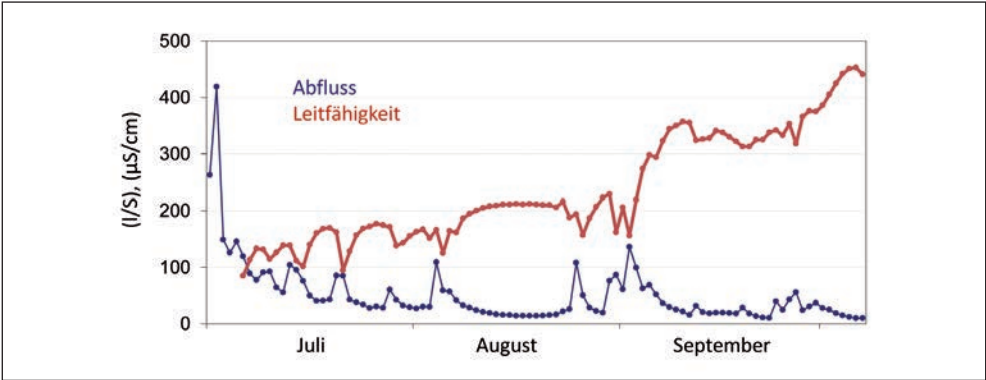
Abb. 6: Mittlerer Tagesabfluss ( \text{l}/\text{s} ) und elektrische Leitfähigkeit ( \mu\text{S}/\text{cm} ) am Pegel HD zwischen 1.7. und 7.10.2012
