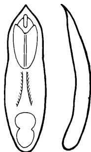
Abb. 2. Phyllotreta tomboi sp. nov. — Aedoeagus des ♂ von unten (a) und von der Seite (b).
