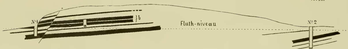
Durchschnitt durch das Braunkohlen-Gebirge von Mutupipi. a. Stollen. b. Kohlenflötz im Abbau. Nr. 1. Schacht. Nr. 2. Schacht.
