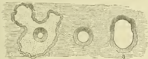
Die Puas von Tokanu am Taupo-See.
