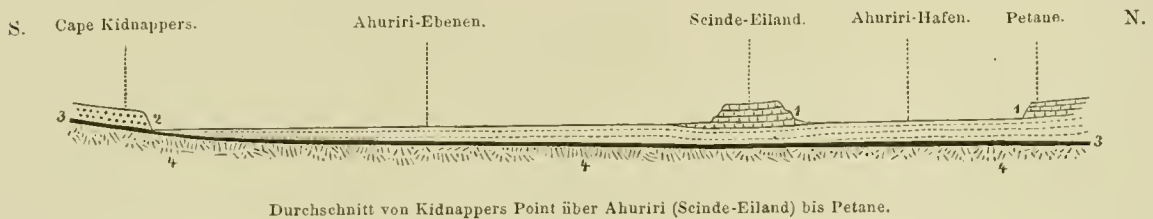
Durchschnitt von Kidnappers Point über Ahuriri (Seinde-Eiland) bis Petane.
