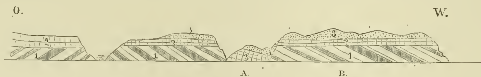
Durchschnitt am Waikato-Southhead.
