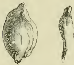
Vulcanische Bomben.
