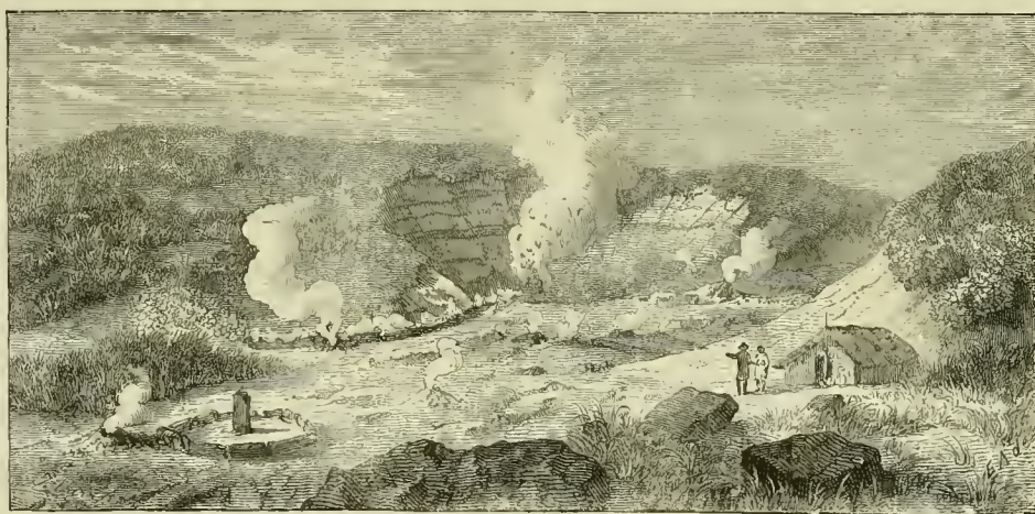
Die Solfatatare Ruahine am See Rotoiti.
