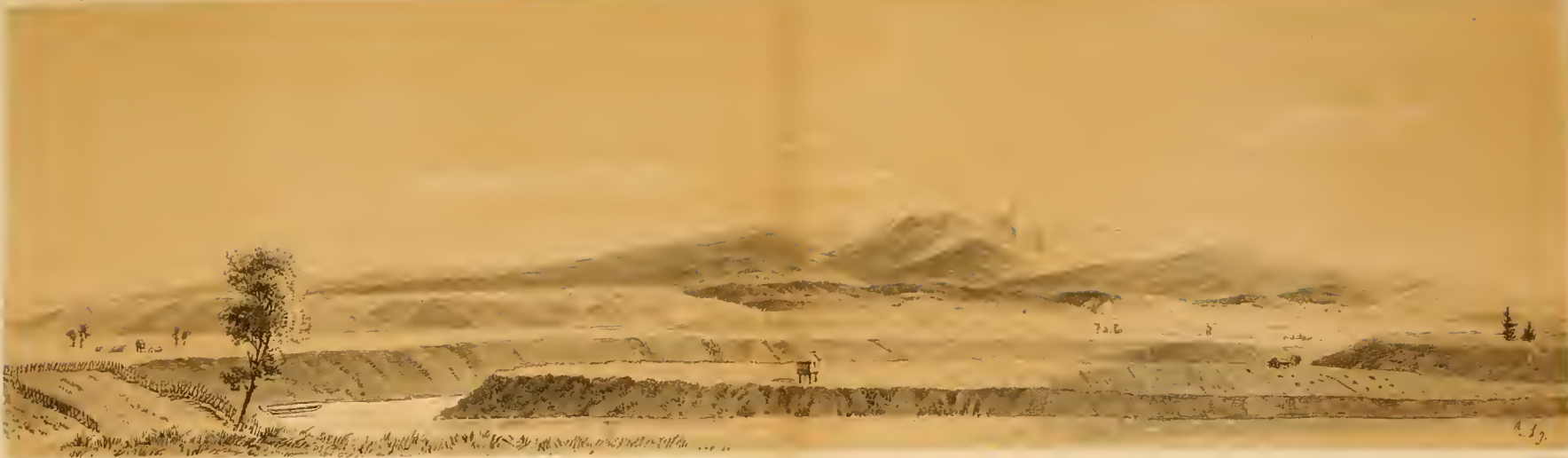
Waiapu Terrassen Pirounga am Waiapu 2630 F von Osten gesehen
