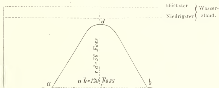
Profil des projectirten künstlichen Rifffes.
