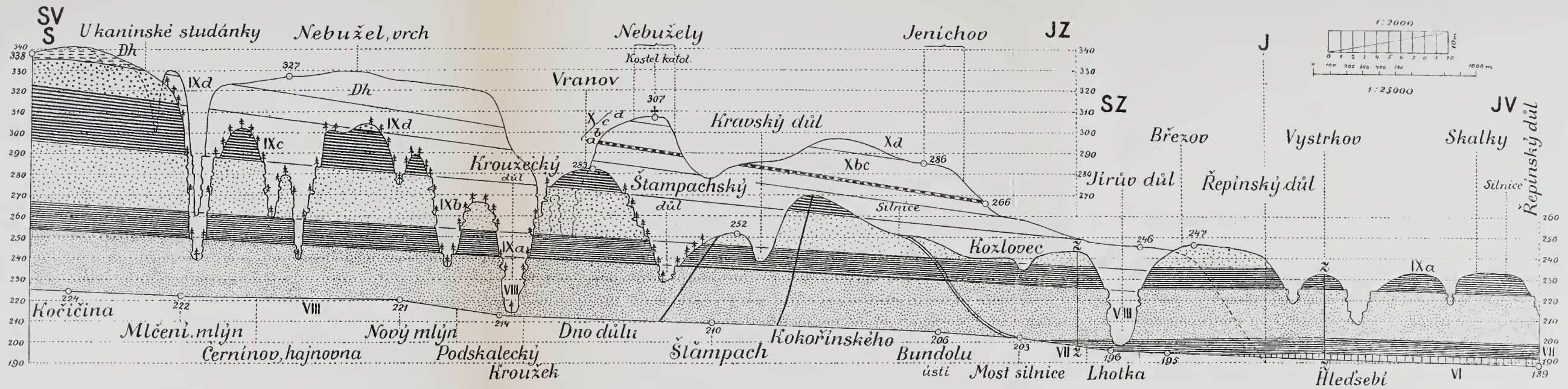
Obr. 52. Nárys levé straně Kokořinského důlu na rovině Kanina (338) Kozlovec, Kozlovec Výstrkov, Výstrkov Šalky a průřez od Kaniny (338) přes Nebužely a Jenichov do Řepinského důlu.
