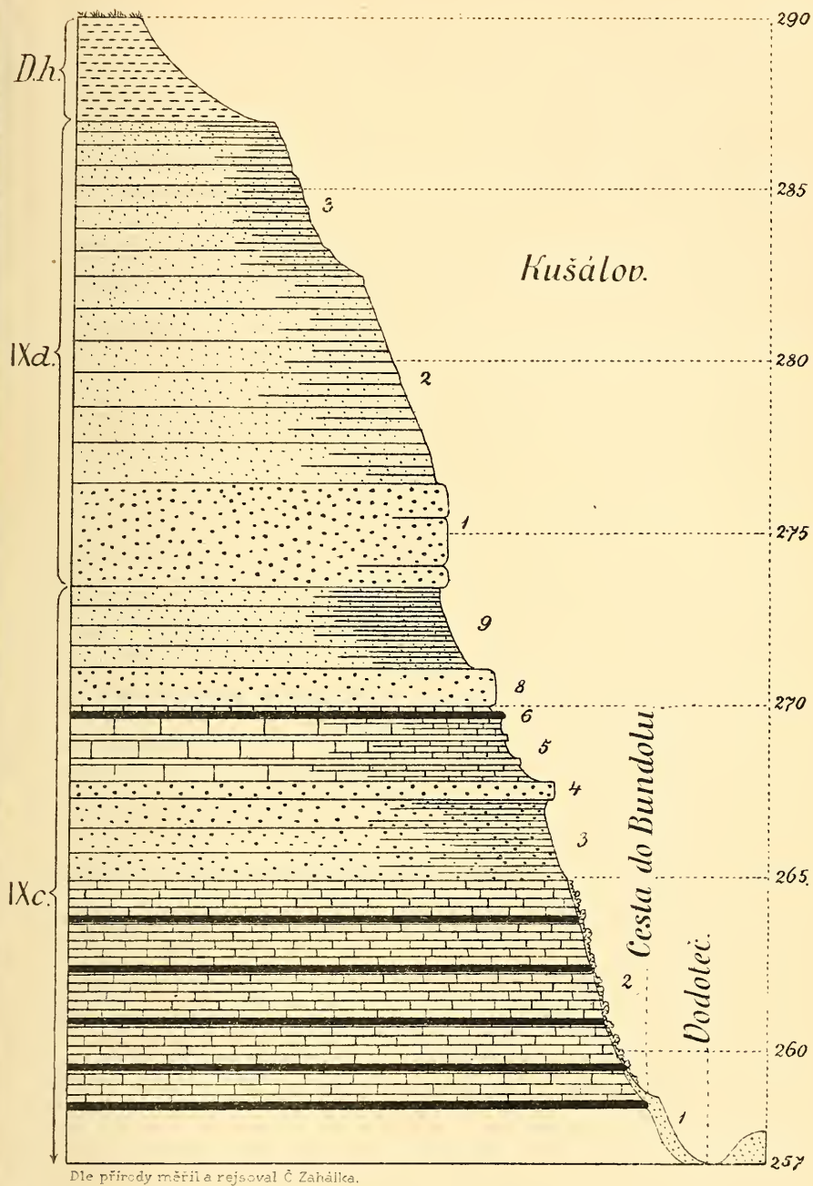
Obr. 50. Průřez strání v Kušálově.
