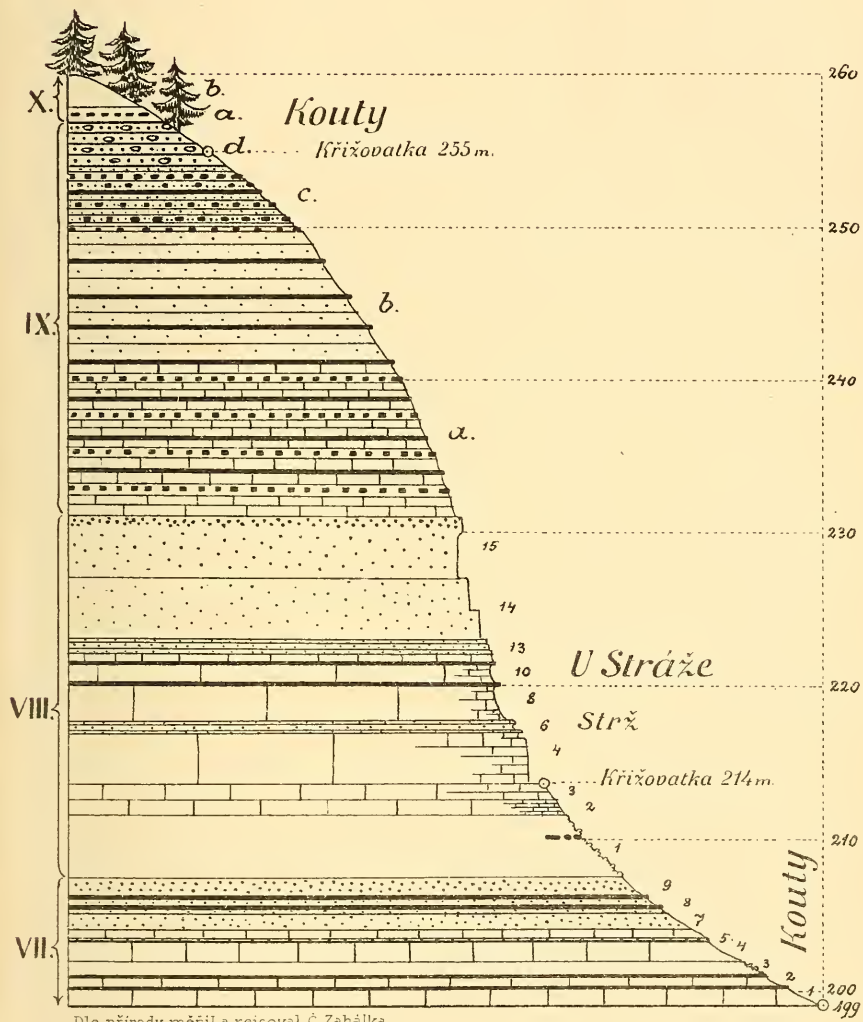
Obr. 44. Průřez dle cesty z Raholin pod Hostlinu.
