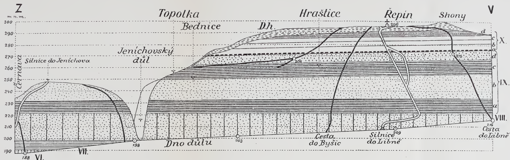
Obr. 48. Narys pravé straně Řepínského důlu na rovině Z.V. Hledsebi-Řepin (Kostel)
