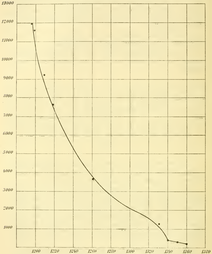
Fig. 6. Labradorit.
