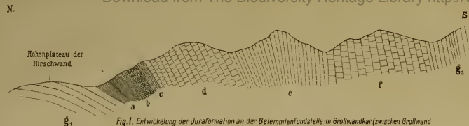
Fig. 1. Entwicklung der Juraformation an der Belemnitenfundstelle im Großwandkar (zwischen Großwand und Pleistigkei, Radstädter Tauern). Oberer Durchschnitt.
