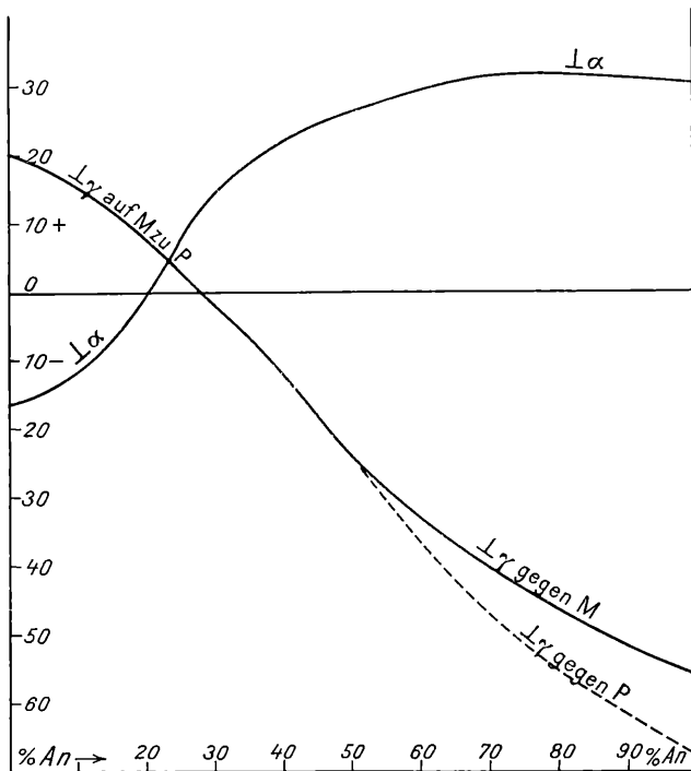
Fig. 1. Auslöschungskurve bei Plagioklassen in Schnitten \perp\alpha und \perp\gamma .
