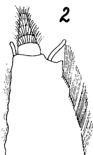
Fig. 2. Trichoniscus chasmatophilus n. sp., ♀. Endabschnitt des Innenastes Maxillarfußes, 485mal.
