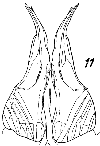
Fig. 11. Chaetophiloscia leucadia n. sp., ♂, 5 mm lg. Fig. 12. Chaetophiloscia leucadia n. sp., ♂, 5 mm lg.
