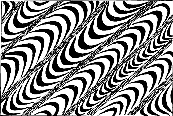
Fig. 2. Zerlegung eines stark einseitig übertriebenen Faltenplanes durch Zerreiung und reihenweise Zusammenschleifung der Mittelschenkel.
