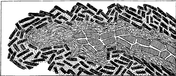
Fig. 4. Schema einer rauhen Stirnfalte, die aus vorher schon tektonisch zerbrochenen und verschieferten Schichten gebildet wurde.
