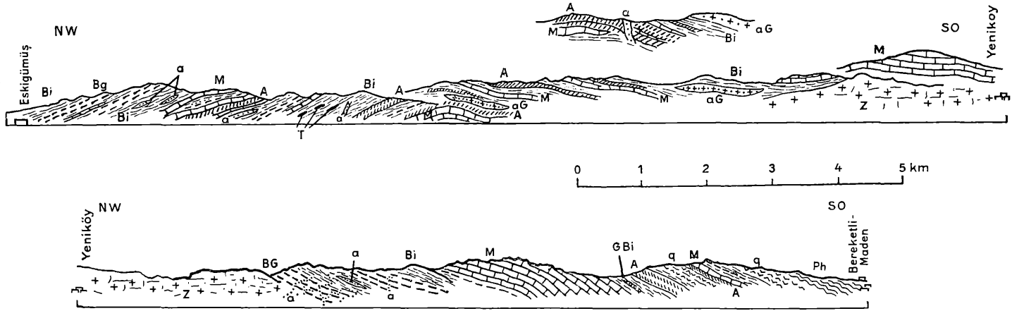
Fig. 9, 9a. Profile durch das Kristallin zwischen Niğde und Bereketli-Maden.
