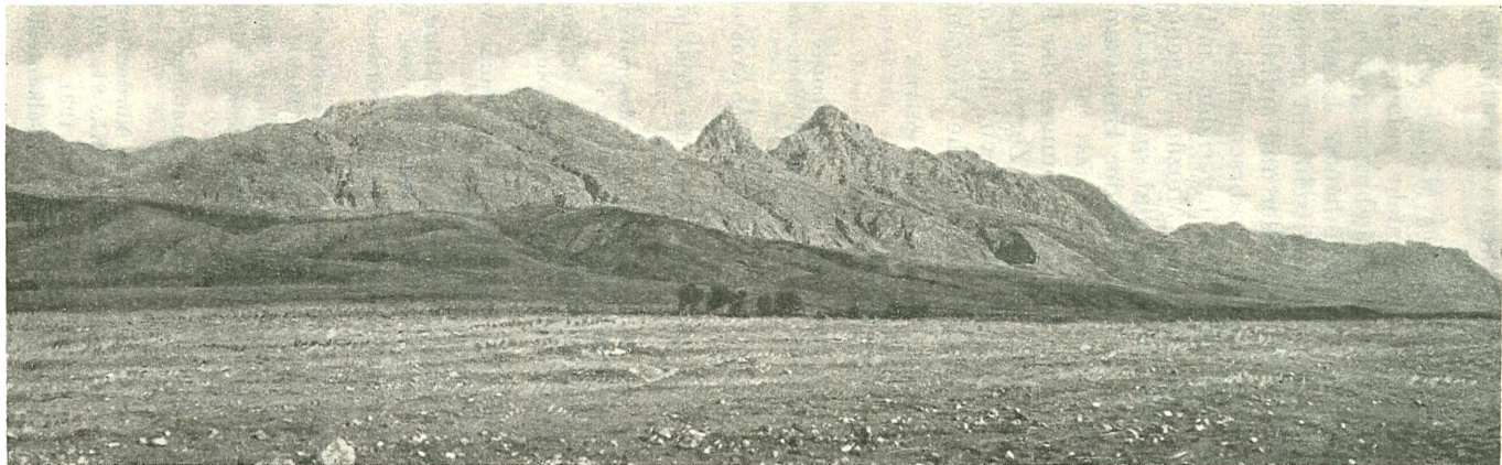
Fig. 12. Der Ala Dagh südlich des Çemistales vom W gesehen. Zentral der große und kleine Demirkazyk. Zu beachten sind die vom S gegen N allmählich ansteigenden Flächensysteme.
