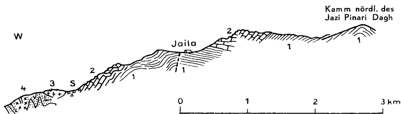
Fig. Profil im nördlichen Ala Dagh.
