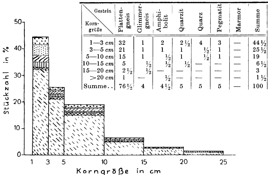
Fig. 2b. Rettenbach, Schotterbank oberhalb der Mündung in die Laßnitz.
