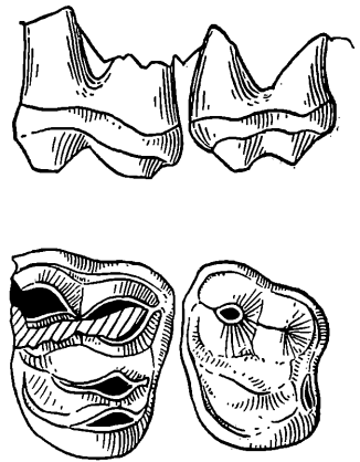
Abb. 13. Hemicyon sansaniensis Lartet. Linker M^1 und M^2 . Seitenansicht und von der Kaufläche. Helvet, Spalte von Neudorf a. d. March. \frac{1}{4} nat. Gr.
