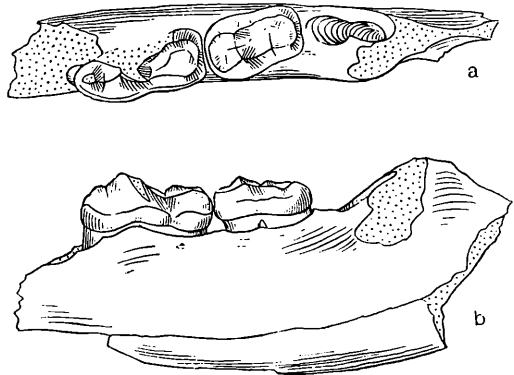
Abb. 14. Ursavus brevirhinus (Hofm.). Linkes Unterkieferbruchstück mit M_1 und M_2 . a) von der Kaufläche, b) Seiten-(Außen-)Ansicht. Helvet, Spalte von Neudorf a. d. March. \frac{1}{2} , nat. Gr.
