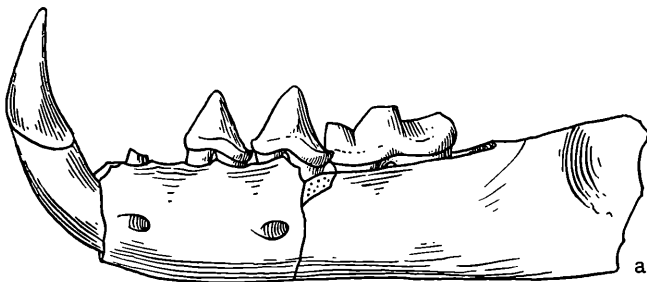
Abb. 2. Trocharion albanense F. M a j. Linker Unterkiefer mit C und P_3 — M_1 . a) Seitenansicht, b) Ansicht von der Kaufläche. Helvet, Spalte von Neudorf a. d. March. \frac{2}{4} nat. Gr.
