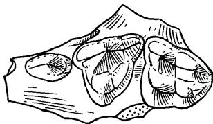
Abb. 1. Trocharion albanense F. M a j. Linkes Oberkieferbruchstück mit P^3 bis M^1 . Seitenansicht und Ansicht von der Kaufläche. Helvet, Spalte von Neudorf an der March. \frac{2}{4} nat. Gr.
