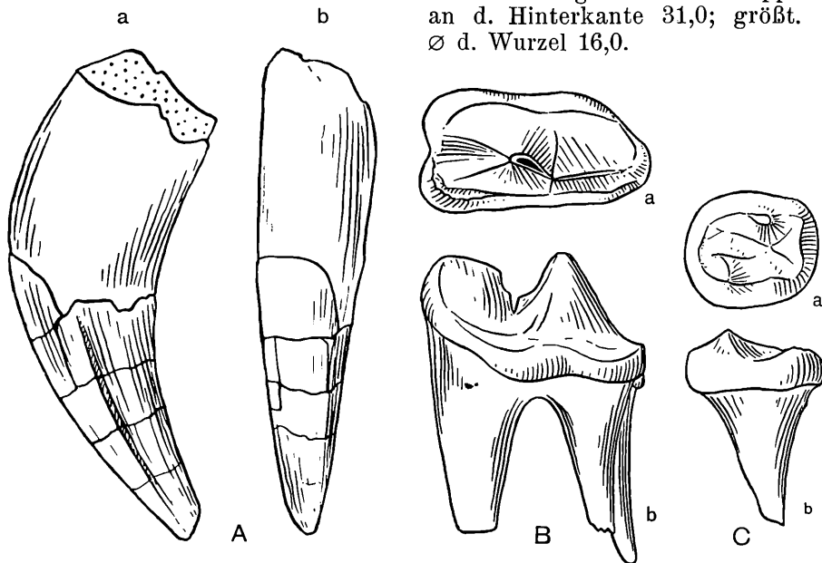
Abb. 10. Amphicyon cf. steinheimensis Fraas. A. Rechter oberer Canin, a) Innen-, b) Vorderansicht; B Linker P 4 , a) von der Kaufläche, b) Seitenansicht; C. Rechter M 3 , a) von der Kaufläche, b) Seitenansicht. Helvet, Spalte von Neudorf a. d. March. Etwa \frac{3}{2} nat. Gr.
