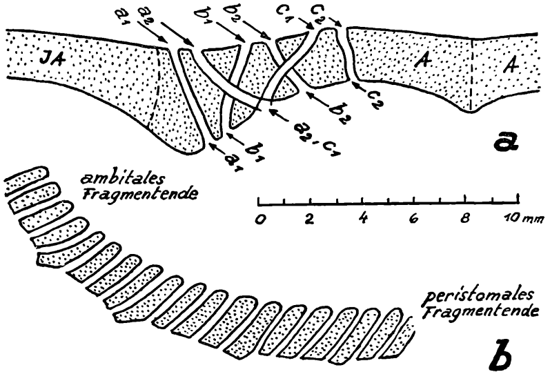
Abb. 3. Porenkanäle von Tripneustes ventricosus austriacus nov. ssp. a) Verlauf der ambulacralen Porenkanäle im horizontalen Schalenquerschnitt. A = Ambulacralplatte, IA = Interambulacralplatte. b) Verlauf der ambulacralen Porenkanäle (c 2 ) im medianen Schalenlängsschnitt.
