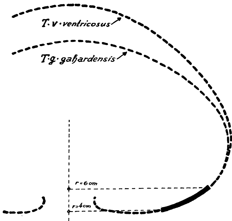
Abb. 2. Rekonstruktion der Lage des Schalenbruchstücks (voll ausgezogen) und der Größe und Gestalt von Tripneustes ventricosus austriacus nov. ssp. — Die beiden dick gestrichelt ausgezogenen Querschnitte repräsentieren etwa die Schwankungsbreite der Gestalt bei verwandten Formen.
