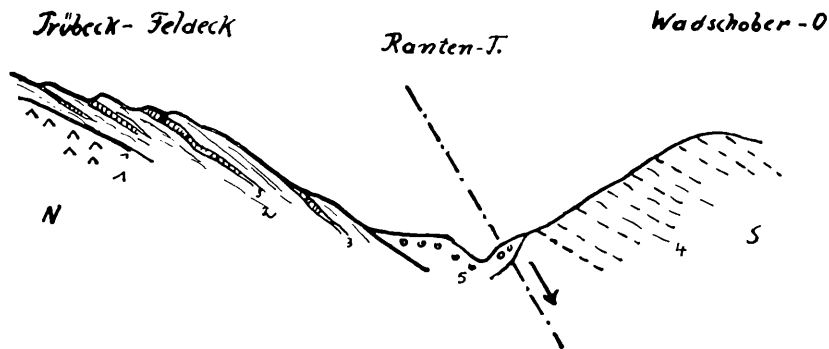
Abb. 4. 1 Granit und Granitgneise; 2 quarzitisches Glimmerschiefer; 3 Amphibolite; 4 Kohlenstoffglimmerschiefer; 5 Schotter (wahrscheinlich diluvial).
