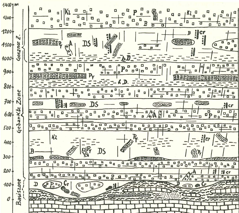
Abb. 1. Der „Radoschatyp“ der Chromerzlagerstätten des Balkanraumes (nach G. Hiebleitner).
