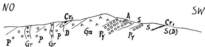
Abb. 2. Der „Ormigliatyp“ der Chromerzlagerstätten im Balkanraum (schematischer Querschnitt durch die basische Zone von Ormiglia auf der Chalkidike, Griechenland).
