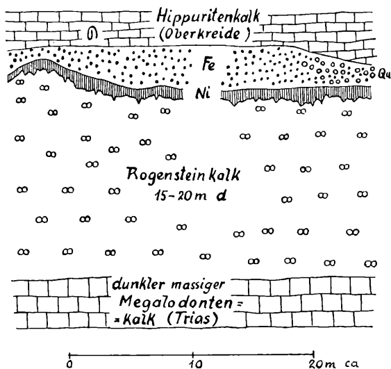
Abb. 4. Nickelerzvorkommen von Marmeko bei Larymna.
