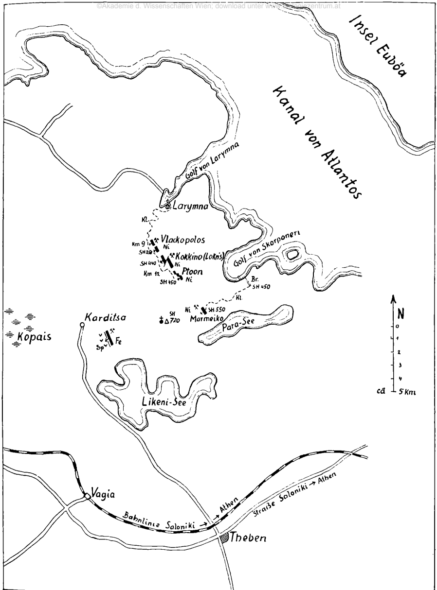
Abb. 3. Übersicht der Nickelerzvorkommen im Norden von Theben (Mittelgriechenland).
