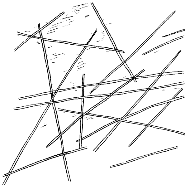
Abb. 6. Venus sp. rez. 650× mit Bohrungen von cf. Ostracoblabe .
