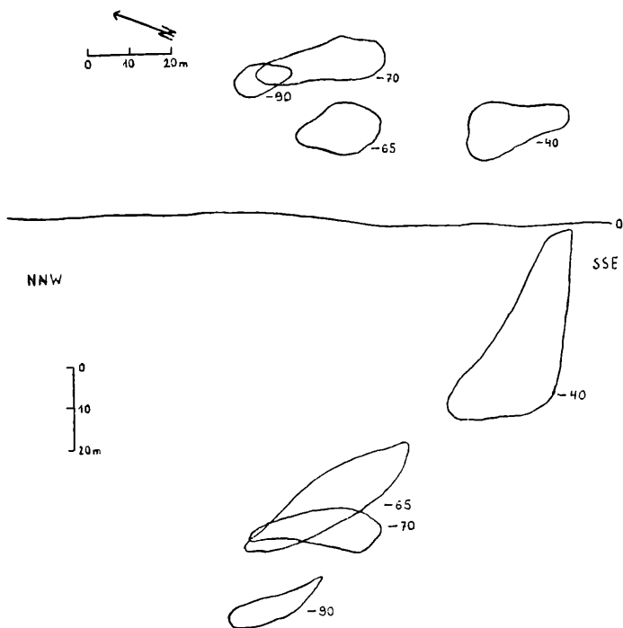
Abb. 4. Grundriß und Schnitt durch die bisher bekannten Erzkörper der Grube Basören I. Signaturen wie Abb. 3.
