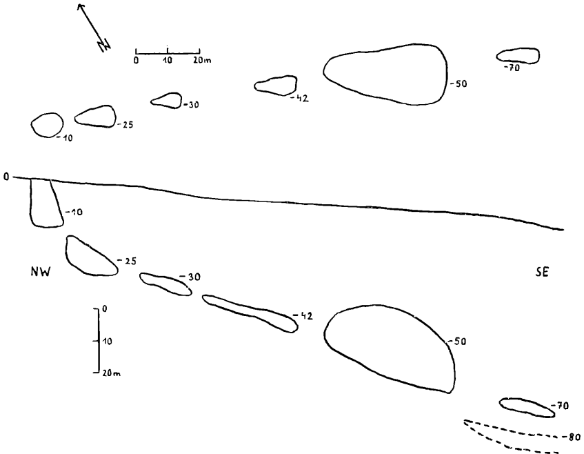
Abb. 3. Grundriß und Schnitt durch die bisher bekannten Erzkörper der Grube Basören II. Voll ausgezogen: Stand der Aufschlußarbeiten im Jahre 1952; strichliert: Stand der Aufschlußarbeiten im Jahre 1954. Nebengestein: Peridotitserpentin.
