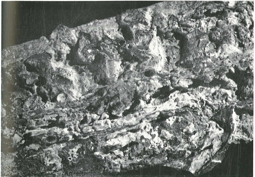
Abb. 2. Teil einer Lanzenspitze (Inv.-Nr. 26016) mit im Brauneisenerz eingebetteten Fannia -Larven, 2 × vergr.
