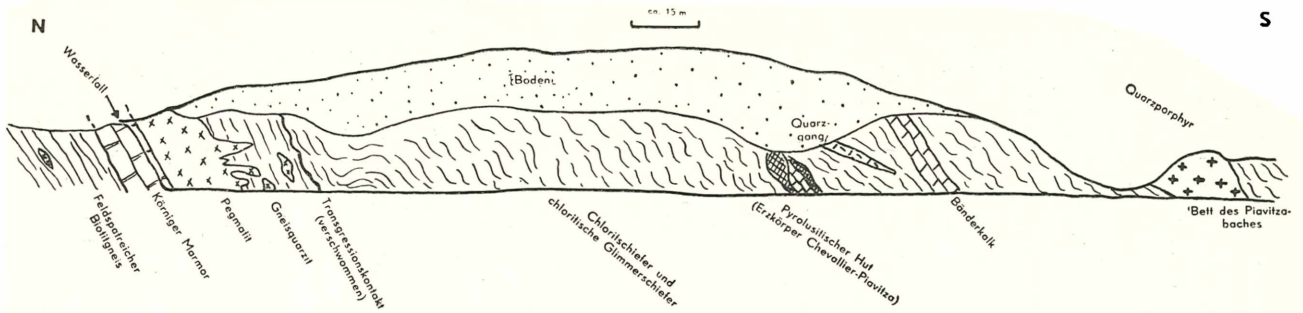
Abb. 5. Geologisches Querprofil entlang dem Oberlauf des Piavitzabaches bei Piavitzta.
