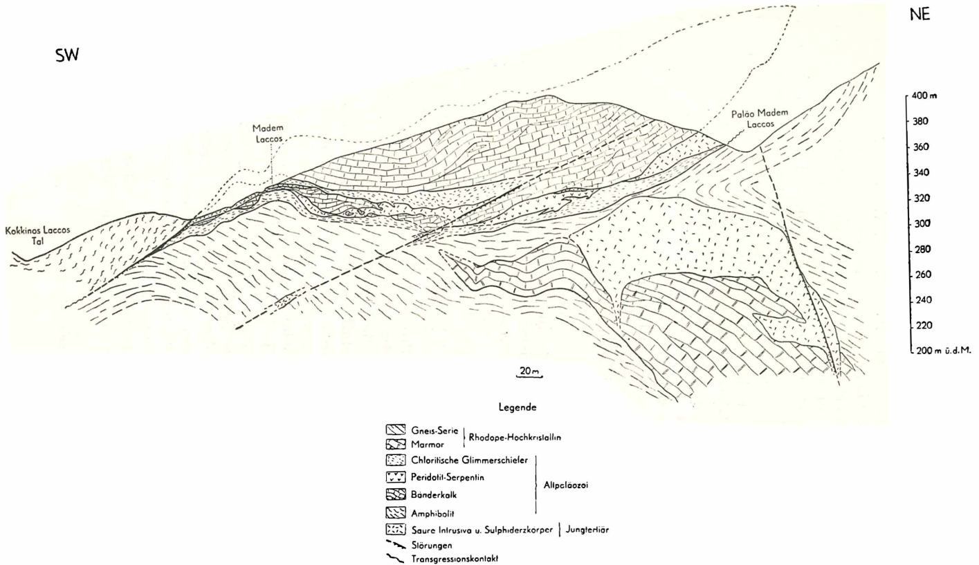
Abb. 1. Querprofil am Rande der Rhodopen bei der Bergbausiedlung Madem Laccos westlich von Stratonii.
