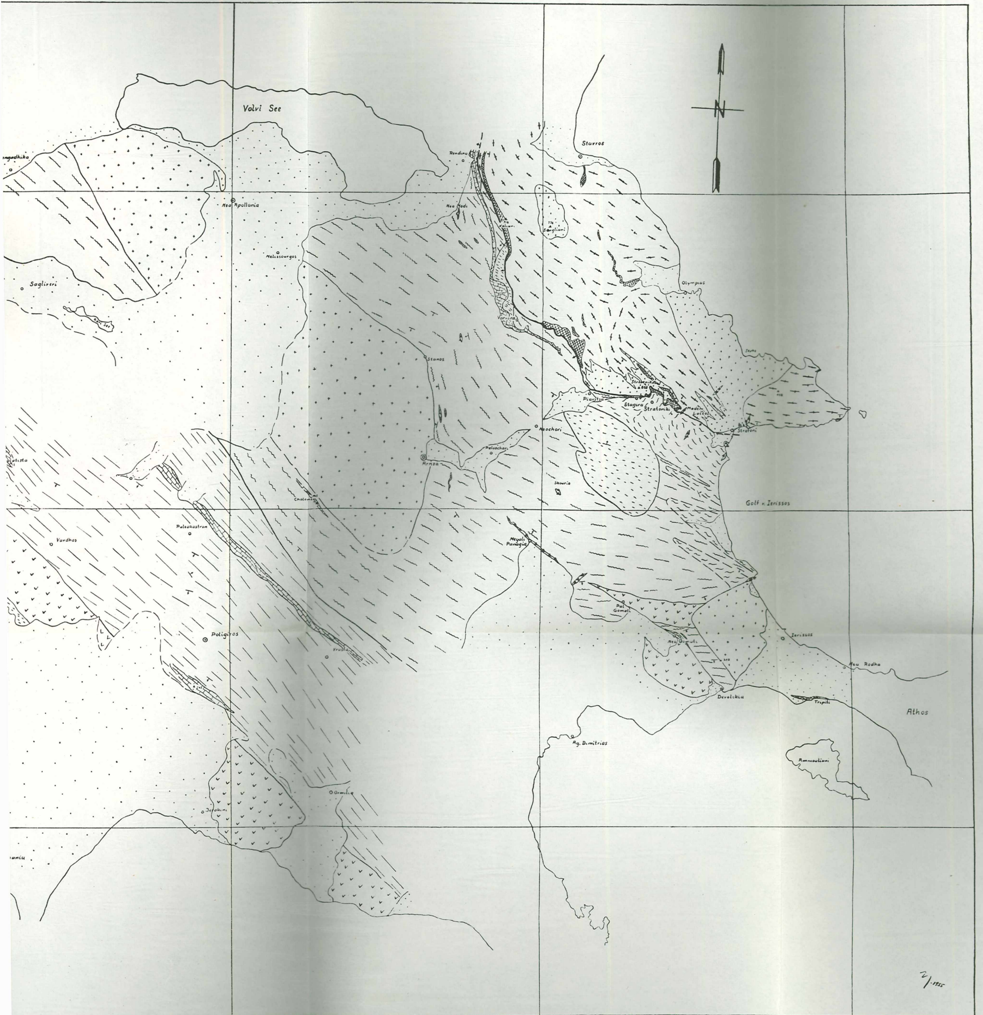
Geologische Karte der Chalkidike. Entworfen nach geologischen Aufnahmen von W. H. Neubauer unter Benützung der Übersichtskarte von G. Hießeleitner und E. Clar.
