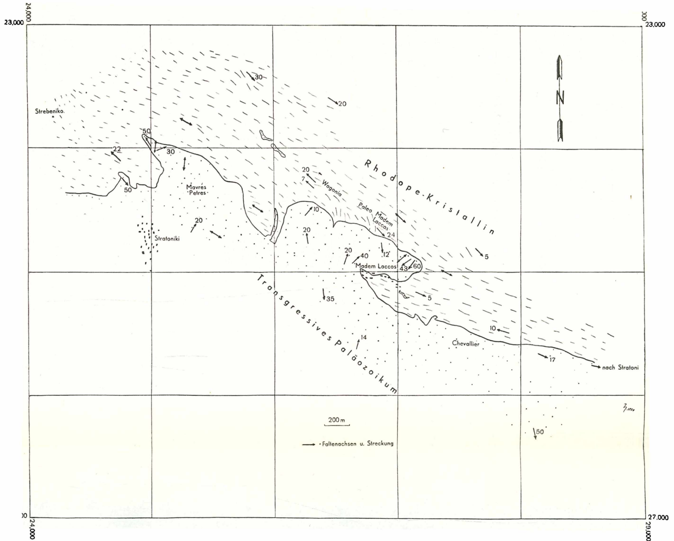
Abb. 2. Karte der B-Achsendiskordanz im Raum Straton-Stratoniki.
