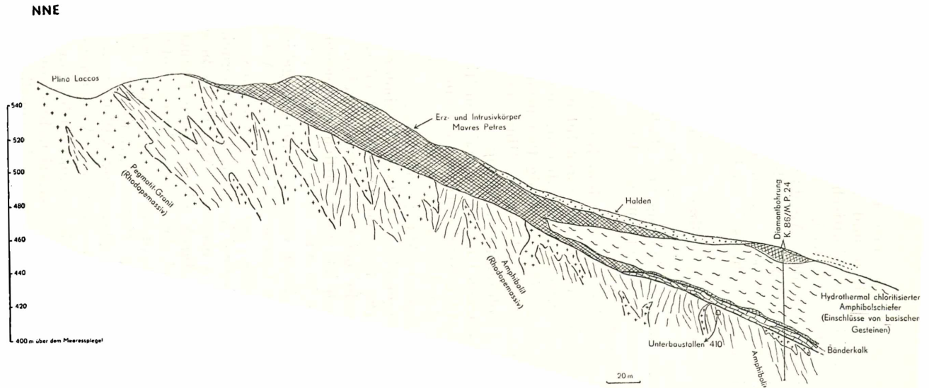
Abb. 3. Querprofil durch die Schichtendiskordanz bei Mavres Petres östlich von Stratoniki.
