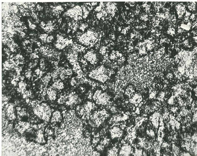
Abb. 6: Blaugrauer Kalk mit braungelben Dolomiteinlagerungen, Gr. 71: Man unterscheidet leicht die überaus feinen Kalkspatgewebepartien gegenüber den groben, idiomorphischen Dolomitgewebeteilen, in denen einzelne Körner eine unvollkommene Rhomboederentwicklung zeigen. Wachstumserscheinung, nicht Deformation. Vgl. Text S. 830. Vergr.: 48fach.
