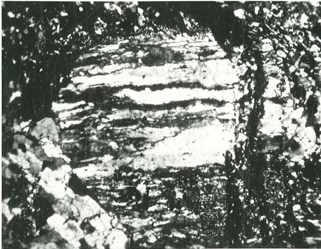
Abb. 2: Graulila farbige Bresche, Gr. 7 (Gerölle). Quarzkorn mit starker transversaler Zerschering als Geröllkorn erhalten geblieben. Vergr.: 48fach.
