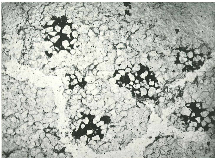
Abb. 3: Zementquarzit, Gr. 49. Beschreibung siehe Text S. 807. Die weißen „Adern“ in der Bildfläche sind nur Schliﬀzerreiungen. Man sieht deutlich sechs der kleinen Gerllchen von resedimentierter Subgrauwacke. Vergr.: 10fach.
