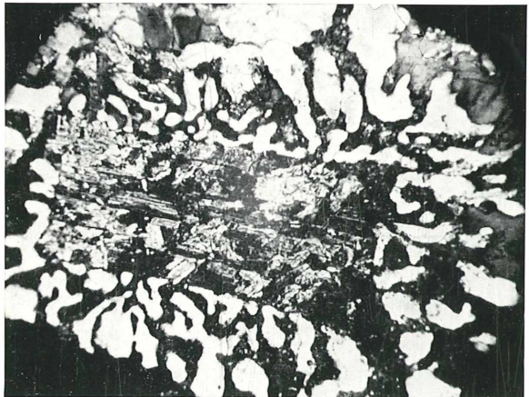
Abb. 5. Granit von Stubenberg (Oststeiermark). — Mikropegmatit. Man sieht im Zentrum einen kristallographisch gut begrenzten KNaF-Kern mit verhältnismäßig groben Muskowiteinschlüssen und sein Weiterwachsen in eine dicke optisch gleich orientierte Rinde, in welcher die schriftzeichenähnlichen Quarze eingewachsen sind. Erklärung: Das zentrale Korn ist ein verdrängter Plagioklas, von dem die Glimmerfülle, welche man im intakten Plagioklas des Gesteins noch sieht, vergrößert erhalten geblieben ist. Der Rand dürfte teilweise aufgezehrtes Quarzkorngewebe sein, das ursprünglich den ehemaligen Plagioklas umschlossen hat. Dafür spricht der Umstand, daß die Quarzstengel felderweise optisch verschieden orientiert sind. Gesamtlänge 2,1 mm. Nic. +
