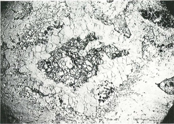
Abb. 2. Massiger Hornblendegabbro (Gerölle), TAGGER, Hönigthal. — Im Kern Olivinreliktkörner, kataklastisch zerlegt, umwachsen von feinkörniger blaßgrüner Hornblende, die nach außen in eine Diablastik mit Plagioklas übergeht. Gew. Licht. Vergr. 16fach.
