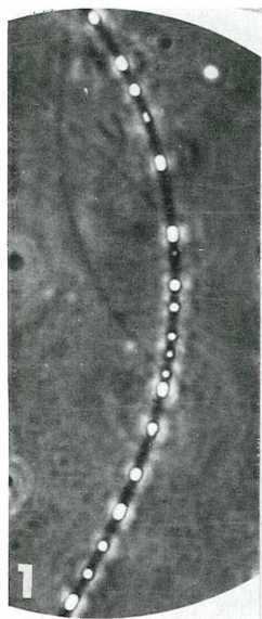
1: Faden von Thiothrix tenuissima , Austritt I/26, Phasenkontrast, 1600fach. — 2: Rundliche Gebilde tierischer Herkunft (enzystierte Protozoen?) vom Austritt I/12, 640fach. — 3: Schwarzfärbung der Schwefeltröpfchen von Thiobacterium bovista des Austrittes I/27a nach Einwirkung von Silbernitrat, 240fach.
