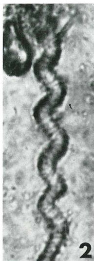
1: Gallionella scheminzkyi , 160fach. — 2: Der oberste Teil der nebenan dargestellten Gallionella , 1600 fach; die Wendelbildung des feinen Fadens ist unverkennbar. — 3: Feine, z. T. in Bündeln liegende, zellig unterteilte Fäden von Leptothrix thermalis mit Berlinerblau-Färbung, 640fach.
