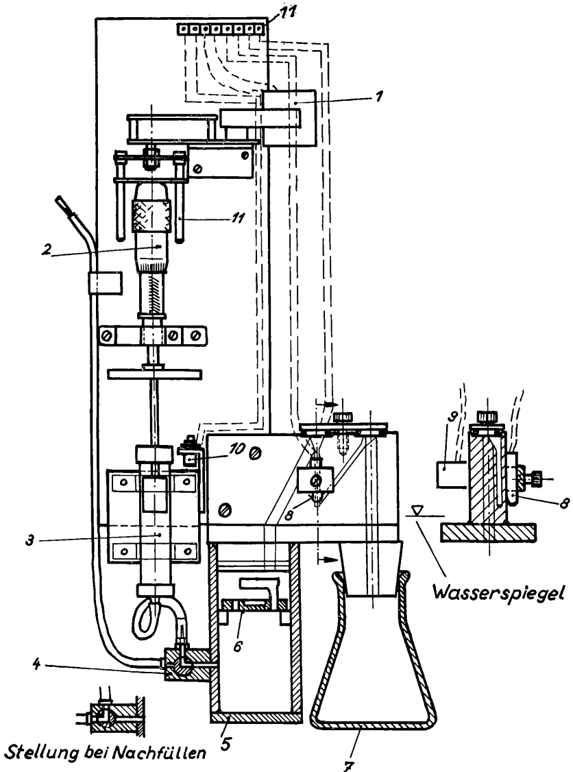
Abb. 1. 1. Motor; 2. Mikrometer; 3. Spritze für Sauerstoff; 4. Umschalthahn zum Füllen der Spritze; 5. Meßgefäß; 6. Behälter für KOH; 7. Ausgleichgefäß; 8. Foto-widerstand; 9. Lichtquelle für die Lichtschranke; 10. Endausschalter; 11. Säulen-führung; 12. Klemmen für elektrische Anschlüsse.
