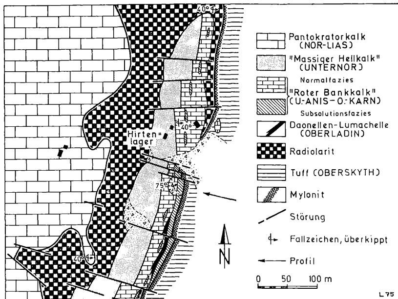
Abb. 2. Geologische Karte der Hallstätterkalk-Scholle von Epidauros (modifiziert nach PELOSIO 1973).
