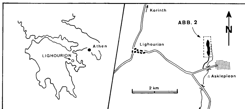
Abb. 1. Lageskizze der Hallstätter Kalke westlich des Asklepieion bei Epidauros.
