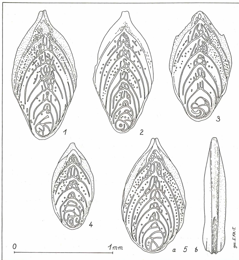
Abb. 5. Neoflabellina ramosa n. sp. Nierentaler Schichten des Untermaastricht des Schweinbachgrabens und des Obermaastricht des Happelgrabensystems E Gams im Gamser Gosaubecken, Steiermark (siehe Abb. 1–2).
