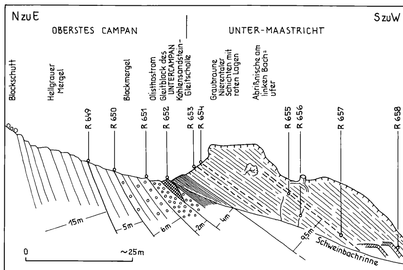
Abb. 2. Profilstück des Schweinbachgrabens NE vom Sommerauer Hof 4,1 km östlich von Gams/Steiermark, den Campan/Maastrichtgrenzabschnitt unterhalb von 800 m Seehöhe mit den erwähnten Mikrofossilfundpunkten zeigend.
