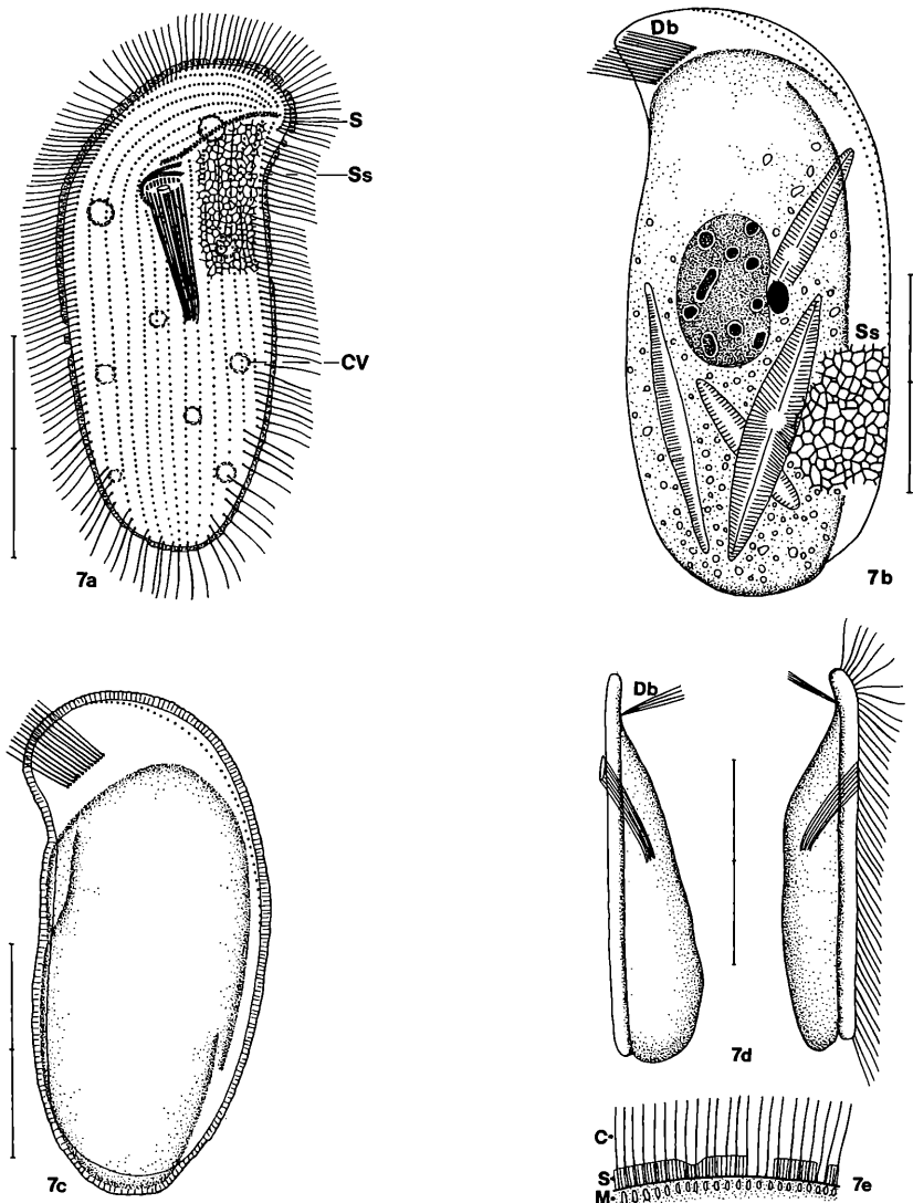
Abb. 7a–e: Trithigmostoma pituitosum nach Lebendbeobachtungen, Infraciliatur und Silberliniensystem (Ss) nach trockener Silberimprägnation. a: Ventralansicht. CV = kontraktile Vakuole, S = Schleimschicht. Skala 30 \mu\text{m} . b, c: Dorsalansichten. Db = Dorsalbürste. Skala 30 bzw. 35 \mu\text{m} . d: Lateralansichten. Skala 40 \mu\text{m} . e: Proximaler Rand stark vergrößert. C = Cilien, M = Mitochondrien, S = Schleimschicht.
