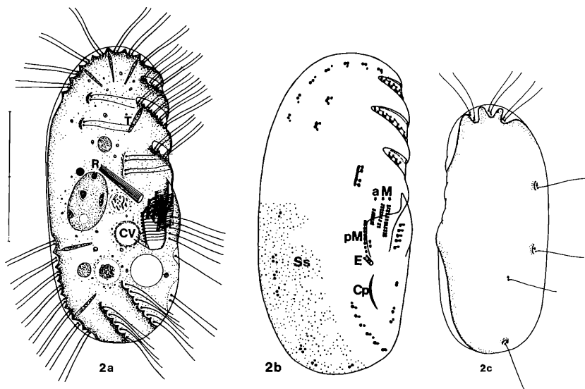
Abb. 2a–c: Drepanomonas sphagni . a: Rechts laterale Ansicht nach Lebendbeobachtungen. CV = kontraktile Vakuole, R = Reuse, T = Trichocyste. Skala 15 \mu m. b: Infraciliatur der rechten Seite und des Oralapparates nach trockener Silberimprägnation. aM = adorale Membranellen, Cp = Cytopyge, E = Exkretionsporus, pM = parorale Membran, Ss = Silberliniensystem. c: Links laterale Ansicht nach Lebendbeobachtungen und trockener Silberimprägnation.
