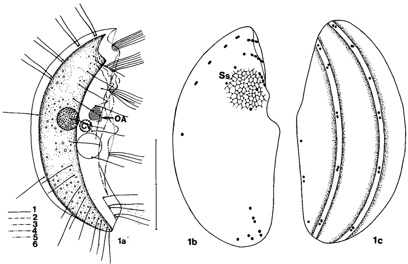
Abb. 1a–c: Drepanomonas lunaris . a: Rechts laterale Ansicht nach Lebendbeobachtungen. CV = kontraktile Vakuole, OA = Oralapparat, 1–6 = Ebenen der Ventralseite. Skala 20 \mu m. b, c: Infraciliatur der rechten und linken Seite. Trockene Silberimprägnation. Ss = Silberliniensystem.
