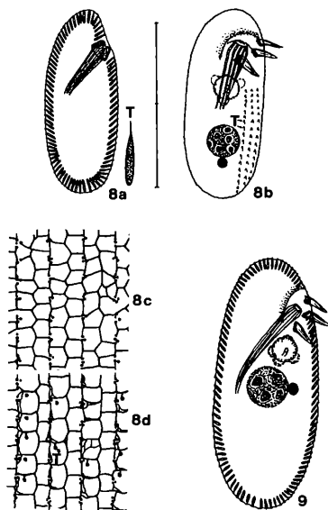
Abb. 8a–d: Furgasonia rubens . a, b: Lateral- und Ventralansicht nach Lebendbeobachtungen. T = Trichocysten. Skala 70 µm. c, d: Silberliniensystem ohne und mit Trichocysten (T). Trockene Silberimprägnation.
