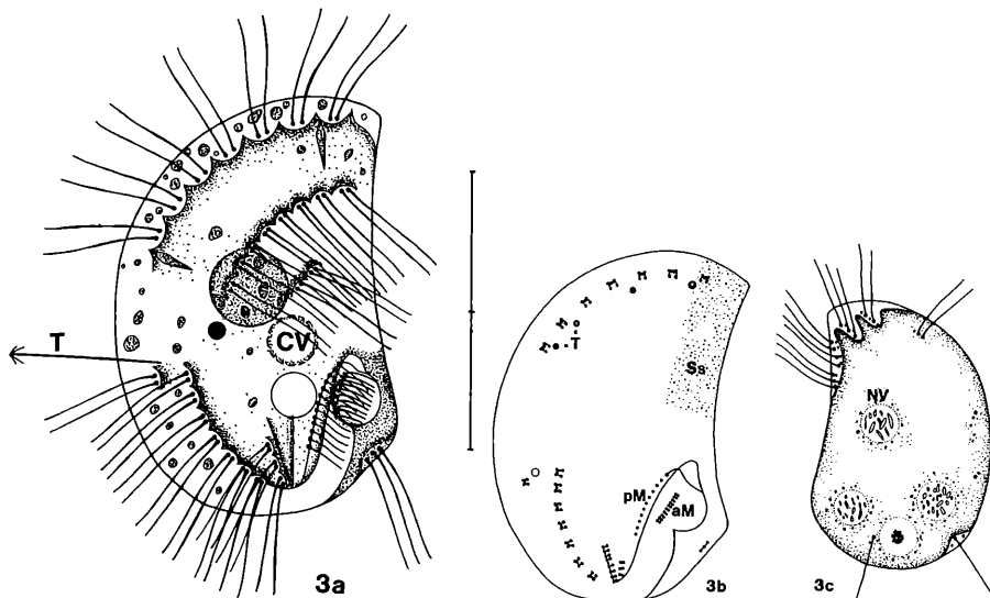
Abb. 3a–c: Microthorax pusillus . a: Rechts laterale Ansicht nach Lebendbeobachtungen. CV = kontraktile Vakuole, T = explodierte Trichocyste. Skala 18 \mu\text{m} . b: Infraciliatur der rechten Seite nach trockener Silberimprägnation und Protargolimprägnation. Körperform nach Lebendbeobachtungen. aM = adorale Membran, pM = parorale Membran, Ss = Silberliniensystem, T = Trichocysten. c: Links laterale Ansicht nach Lebendbeobachtungen und trockener Silberimprägnation. NV = Nahrungsvakuole.
