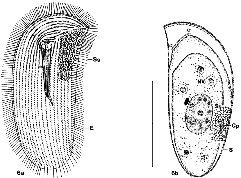
Abb. 6a–b: Trithigmostoma cucullulus nach Lebendbeobachtungen, Infraciliatur nach Protargolimprägnation, Silberliniensystem (Ss) nach trockener Silberimprägnation. Skala 55 \mu\text{m} . a: Ventralansicht. E = Exkretionsporus. b: Dorsalansicht. Die Pfeile weisen auf die Dorsalbürste. Cp = Cytopyge, NV = Nahrungsvakuole, S = Schleimschichte.
