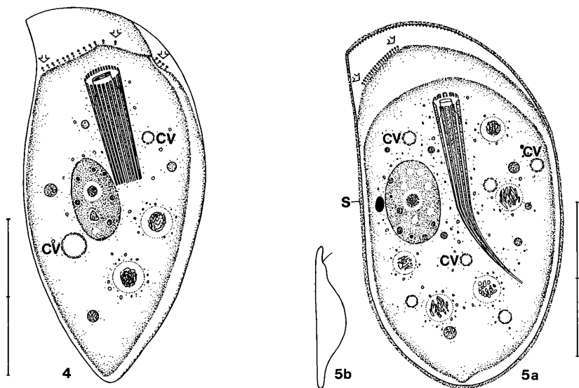
Abb. 4: Pseudochilodonopsis kloiberi . Dorsalansicht nach Lebendbeobachtungen, Dorsalbürste (Pfeile) auch nach trockener Silberimprägnation. CV = kontraktile Vakuole. Skala 30 \mu m.
