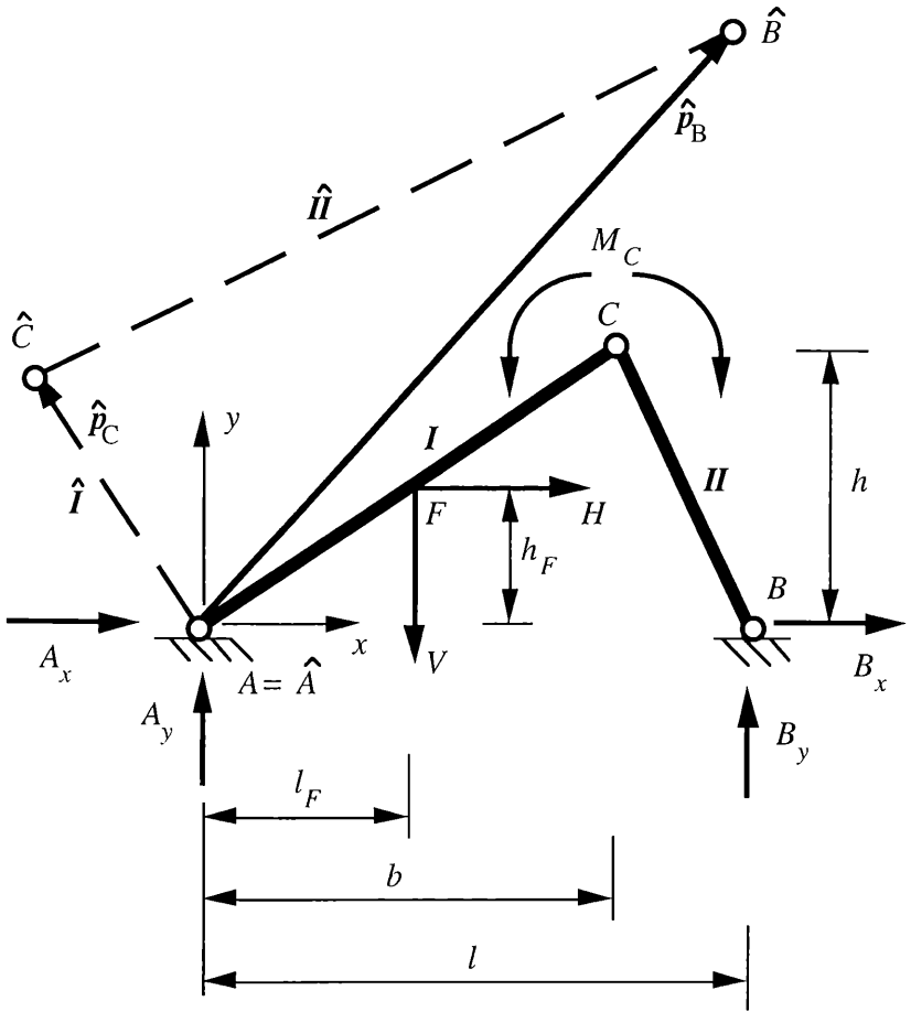
Abb. 1. Dreigelenktragwerk mit Belastung; homogene virtuelle Deformationen nach Gl. (3.14)
