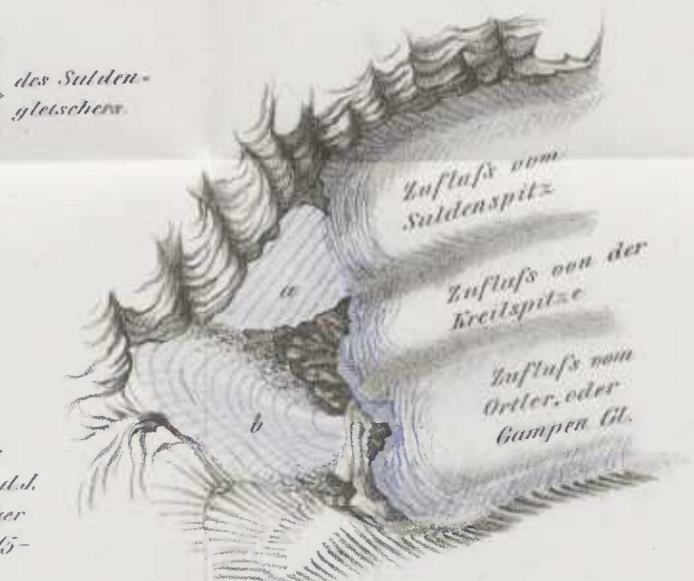
Grundriss des Gletscherendes. a und b der neue Zuwachs. Die blauen Linien zeigen die Lage der Strukturbänder an.
