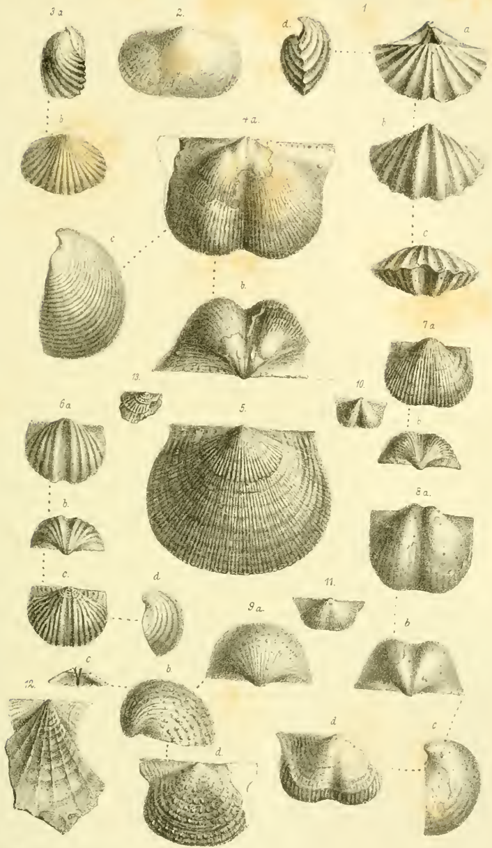
Fig. 1. Spiriferina Hoffriana nov. sp. Fig. 2. Spirifer lineatus Mart. var. ellipticus Son. Fig. 3. Camorpha crumena Mart. sp. Fig. 4. Productus Weyprechti Toula Fig. 5. Productus conf. Prattenianus Norw. Fig. 6. Productus Wilczeki nov. sp. Fig. 7. Productus longispinus Son. Fig. 8. Productus Spitzbergi anus nov. sp. Fig. 9. Productus ( Strophalosia ) Cancrini M. F. R. sp. Fig. 10. Chonetes Verucelliana var. Spitzbergiana n. var. Fig. 11. Chon. granulifera Ov. Fig. 12. Preten Wilczeki nov. sp. Fig. 13. Strophalosia Lophayi Grin.
