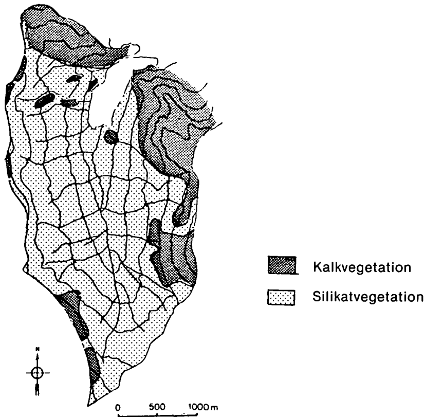
Abb. 2: Verteilung von Kalk- und Silikatvegetation
